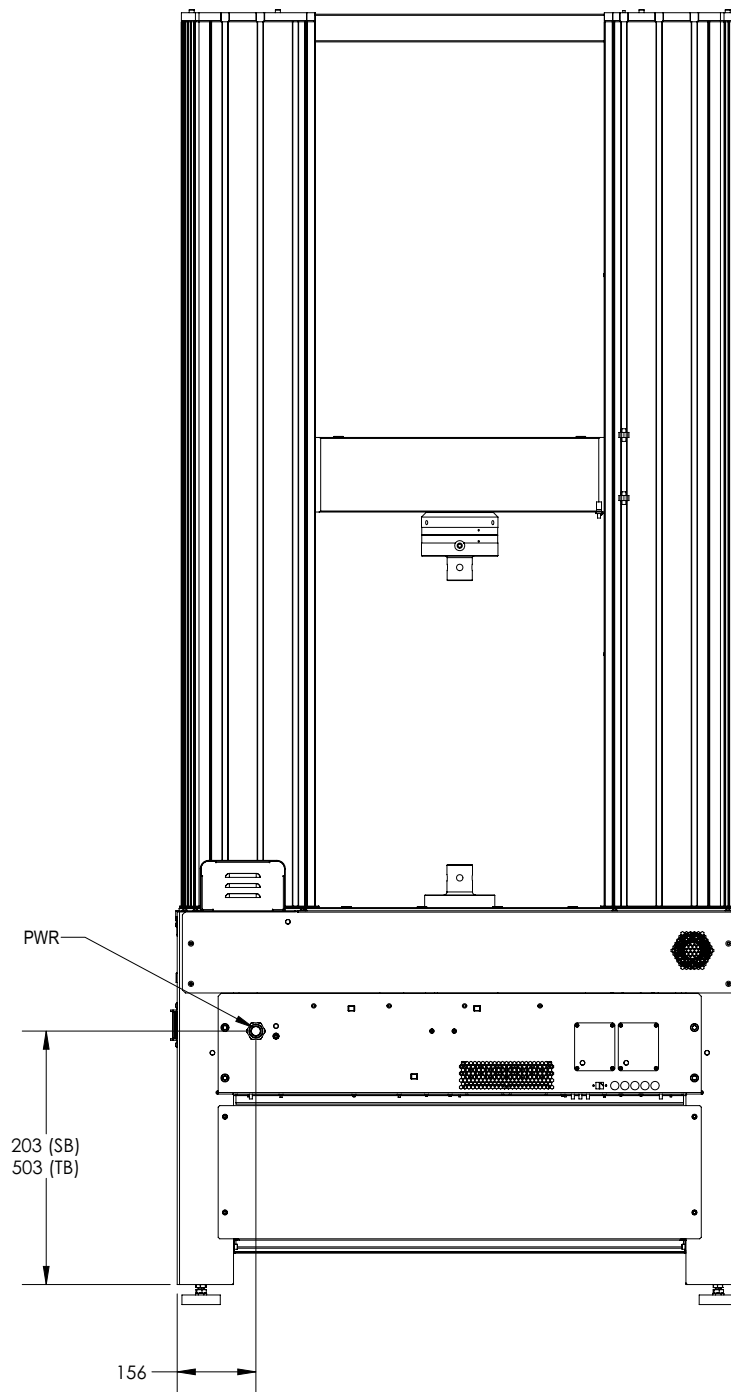
Abbildung 8. 34FM-100 Prüfrahenabmessungen - Rückansicht
