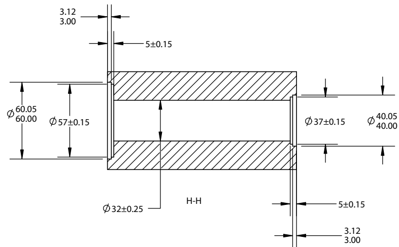
Abbildung 16. Ansicht des Querschnitts H-H der Traverse
