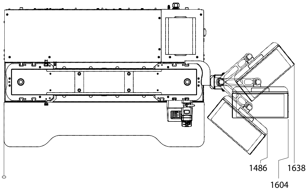
Abbildung 9. 34FM-100 Abmessungen des Rahmens mit Dashboard
