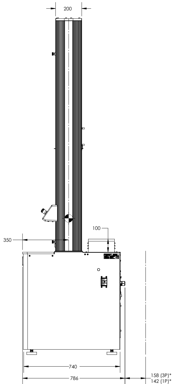
Abbildung 7. 34FM-100 Prüfrahenabmessungen - Seitenansicht
