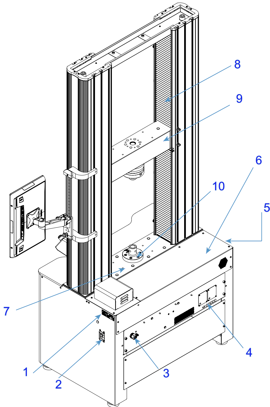
Abbildung 2. 34FM-100 Standmodell mit Bluehill® Bedienerdashboard - Rückansicht
