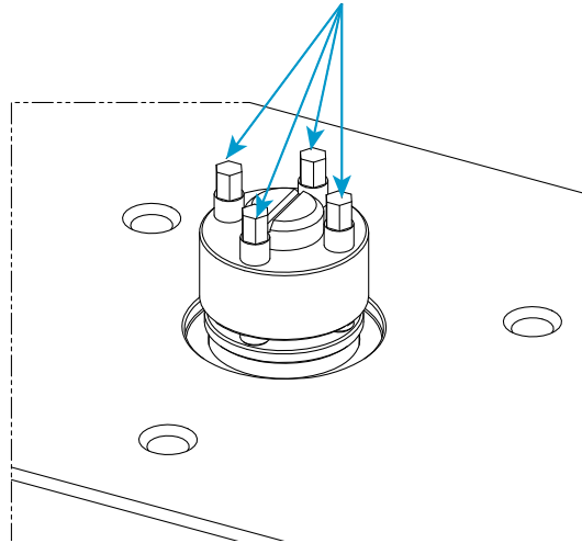
Figura 20. Conjunto de tensor mecánico
