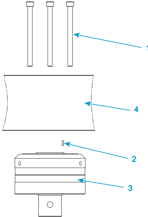
Figura 25. Instalación de una célula de carga de 100 kN de la serie 2530
