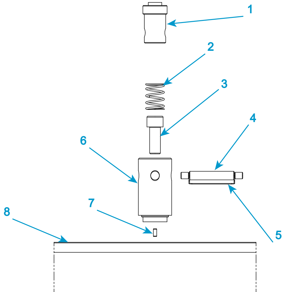
Figura 26. Adaptador de base tipo D
