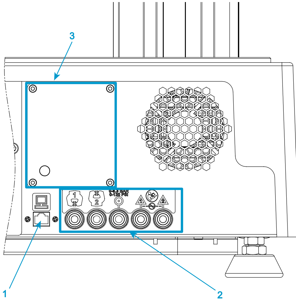
Figura 8. Detalle de conexiones del panel posterior
