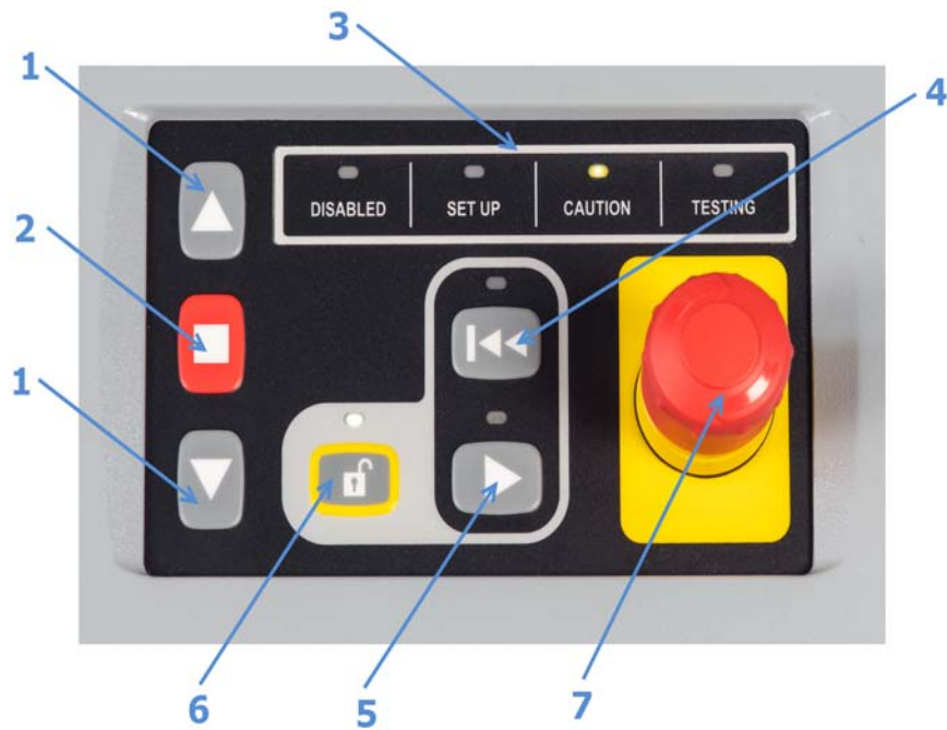
Figura 16. Panel de control del bastidor
