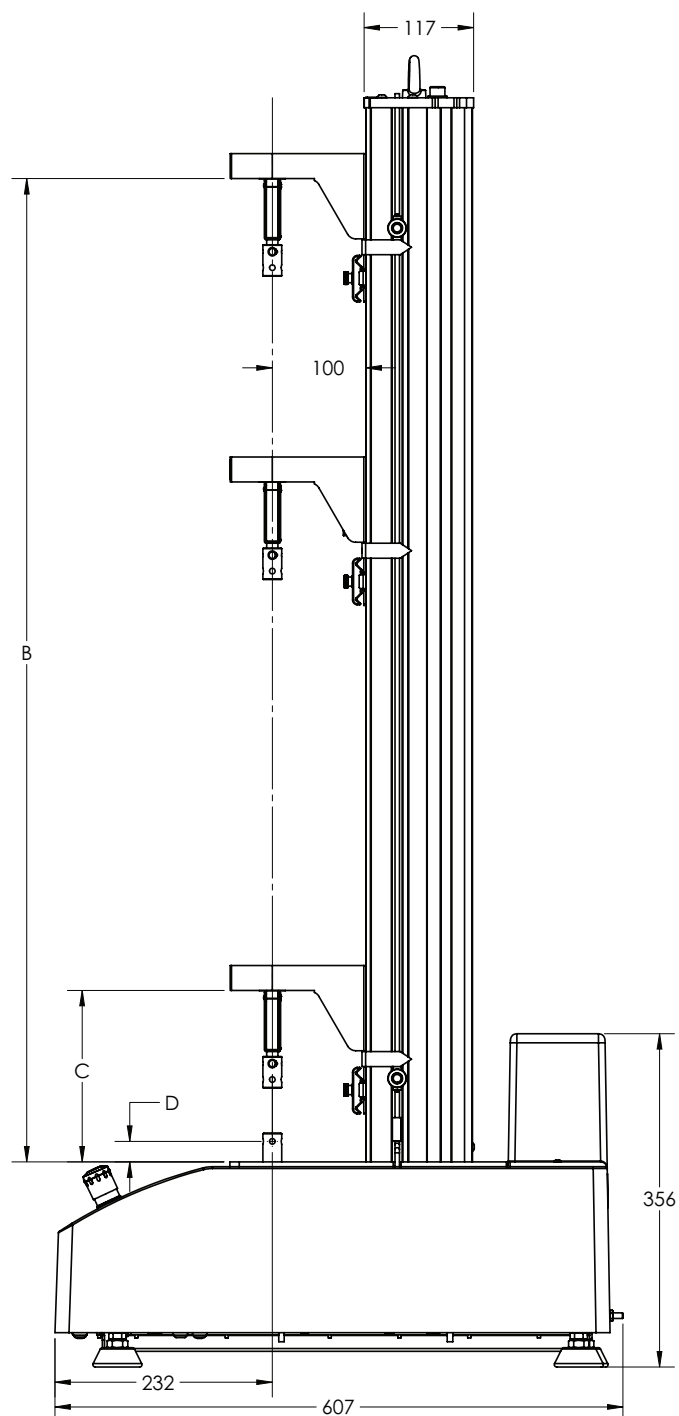
Figura 4. 34SC-5 dimensiones del bastidor: vista lateral
