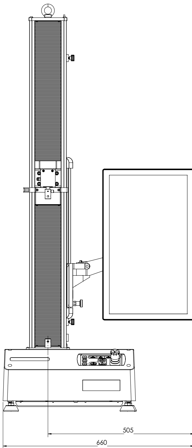
Figura 5. 34SC-5 dimensiones del bastidor, incluida la consola
