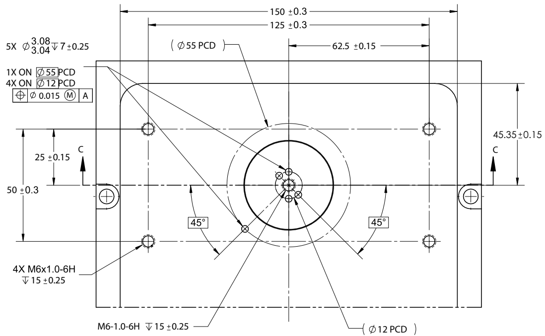
Figura 6. Vista de la ranura de la base desde arriba
