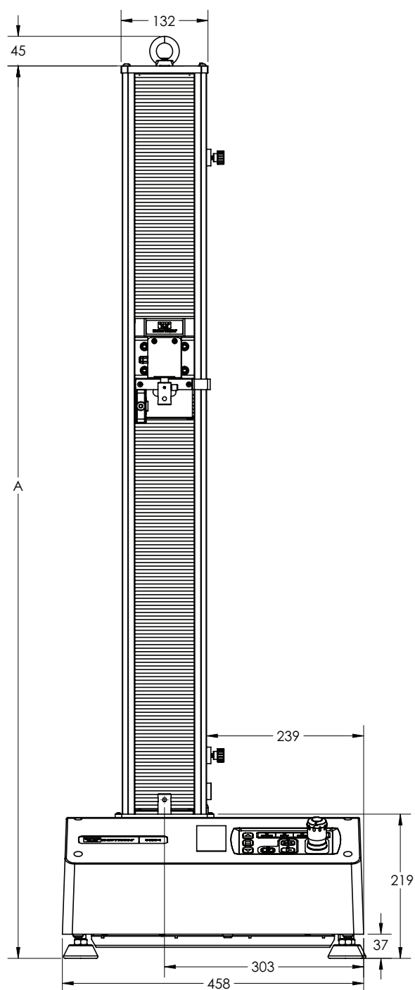
Figura 3. 34SC-5 dimensiones del bastidor: vista delantera
