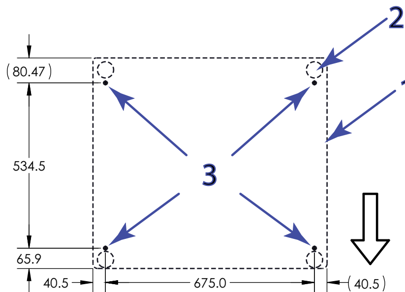
Figura 14. Ubicación de los puntos de anclaje (visto desde arriba)
