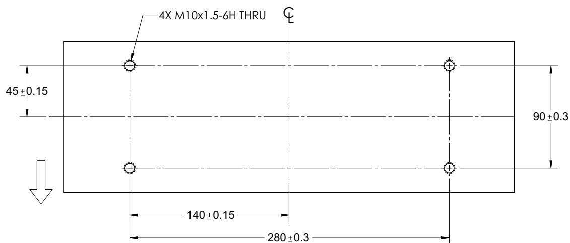
Figura 9. Vista de la parte inferior de la placa superior
