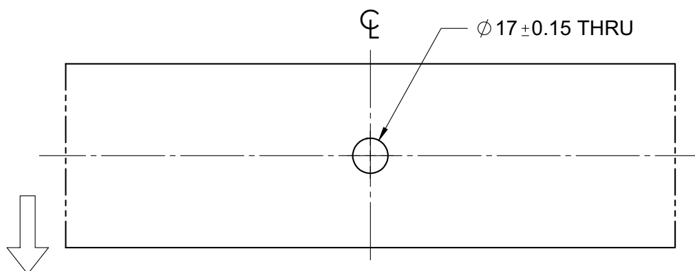
Figura 8. Vista de la parte superior de la cruceta
