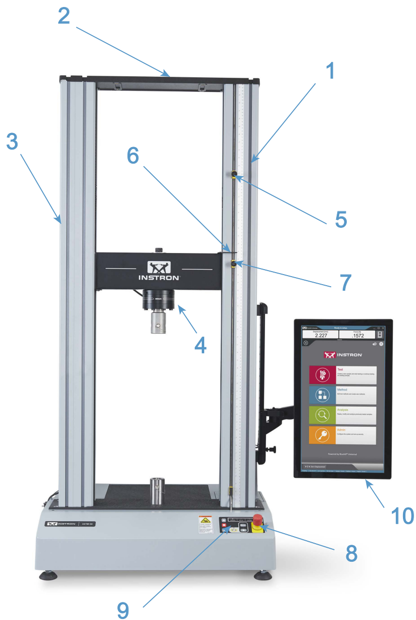
Figura 1. Modelo de sobremesa de dos columnas 3400 con Panel del operador Bluehill® (vista delantera)
