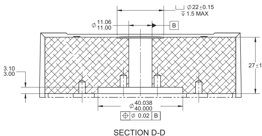
Figura 9. Vista transversal de la cruceta
