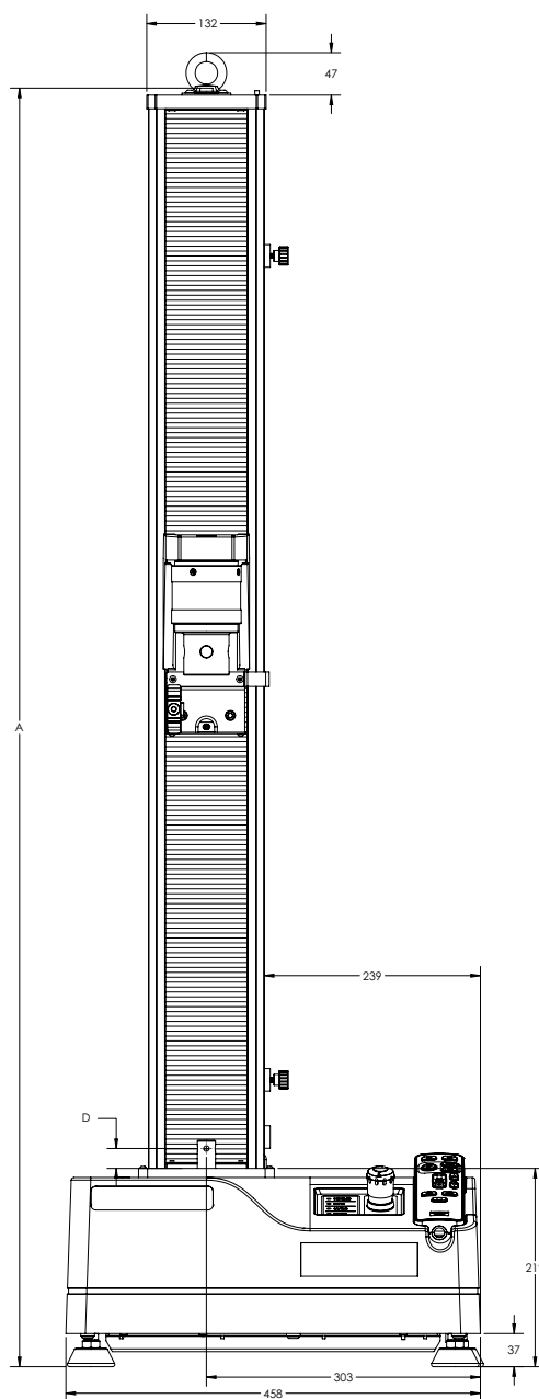
Figura 3. 68SC-5 dimensiones del bastidor: vista delantera
