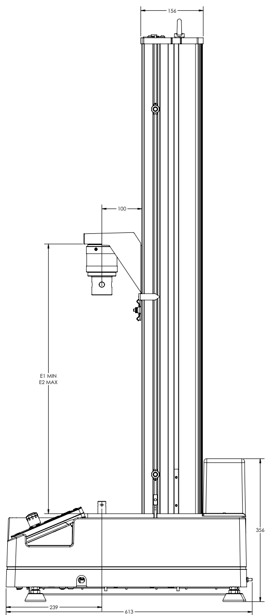
Figura 4. 68SC-5 dimensiones del bastidor: vista lateral
