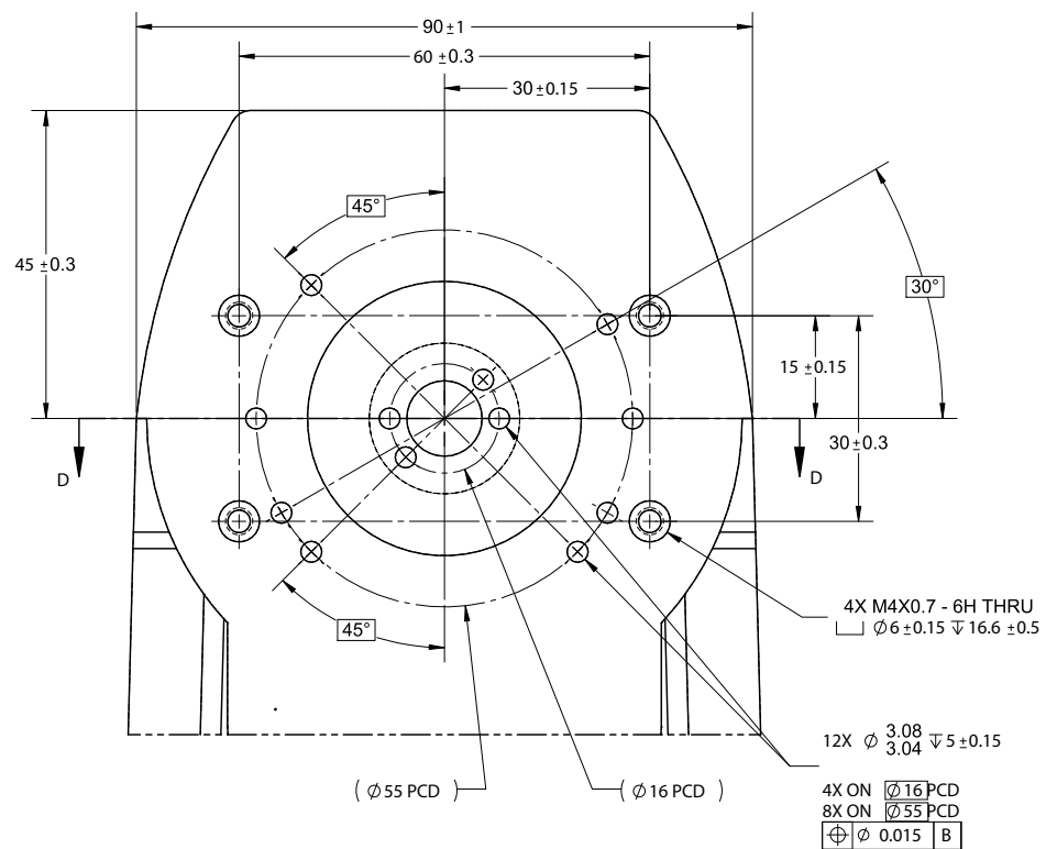
Figura 8. Vista de la parte inferior de la cruceta
