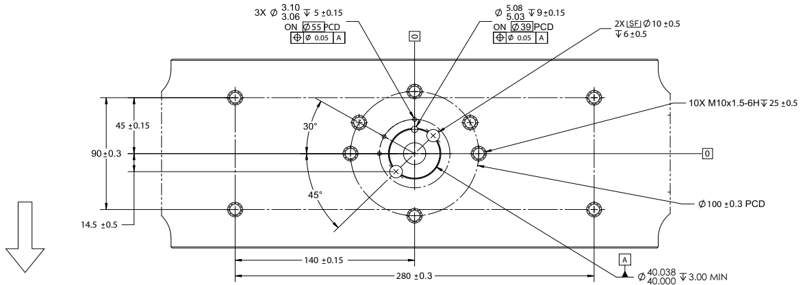
Figura 8. Vista de la parte inferior de la cruceta
