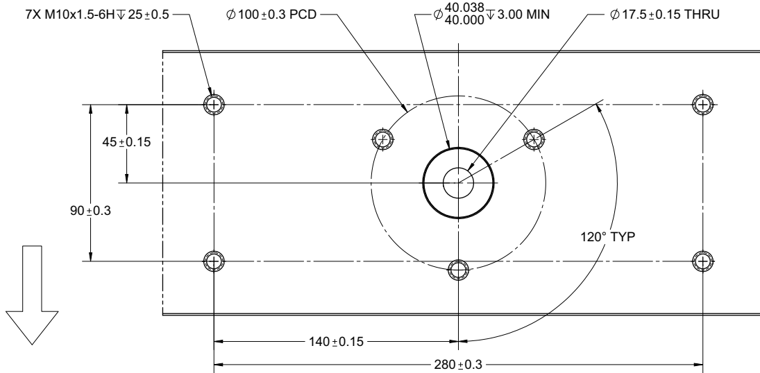
Figura 9. Vista de la parte superior de la cruceta
