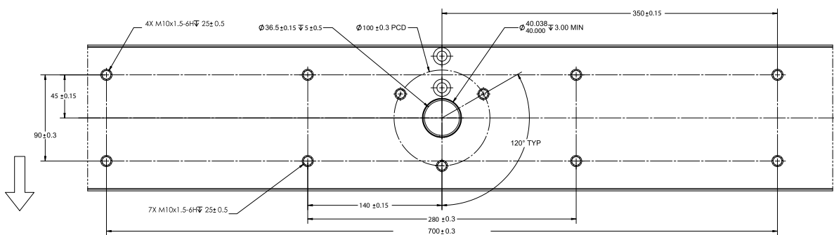
Figura 7. Vista de la ranura de la base desde arriba (solo bastidores de anchura adicional)
