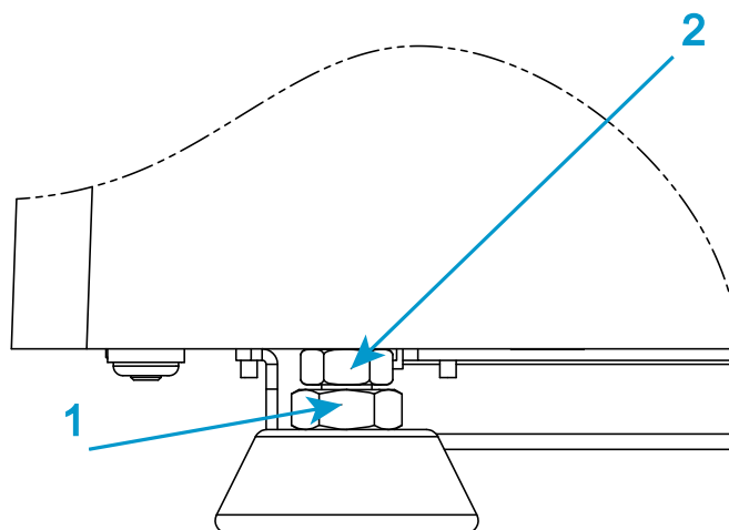
Figura 14. Ajuste de las patas de nivelación
