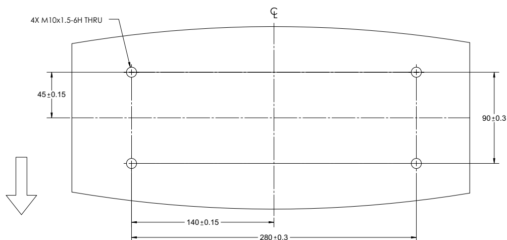
Figura 10. Vista de la parte inferior de la placa superior
