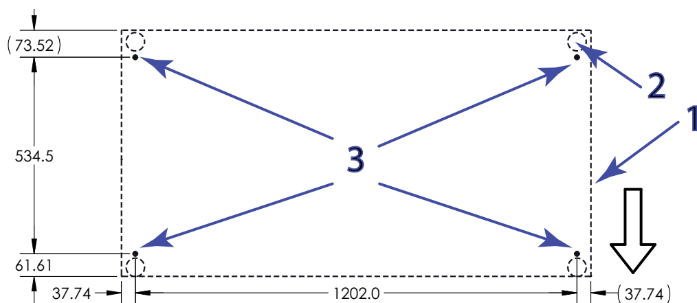
Figura 16. Ubicación de los puntos de anclaje en el bastidor de anchura adicional (visto desde arriba)
