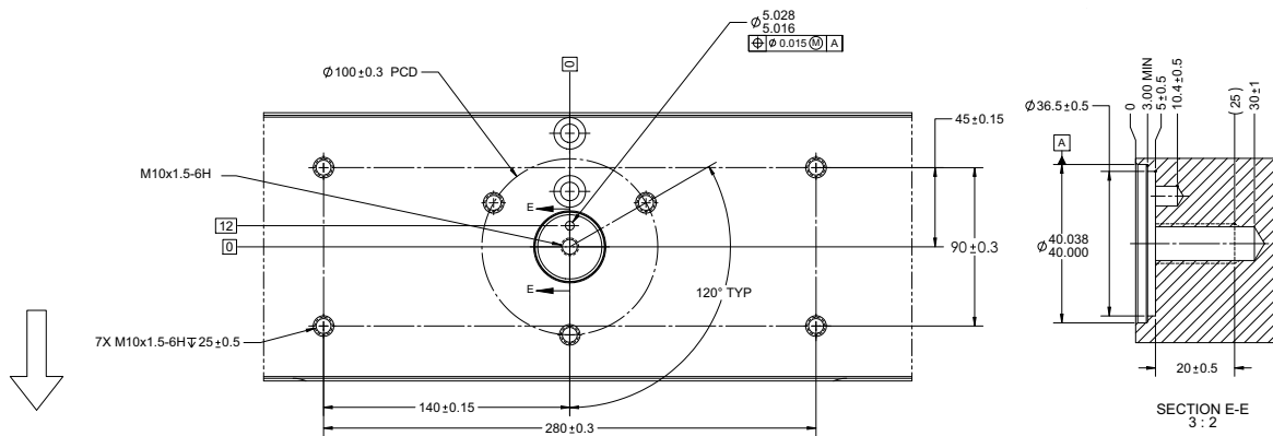
Figura 6. Vista de la ranura de la base desde arriba
