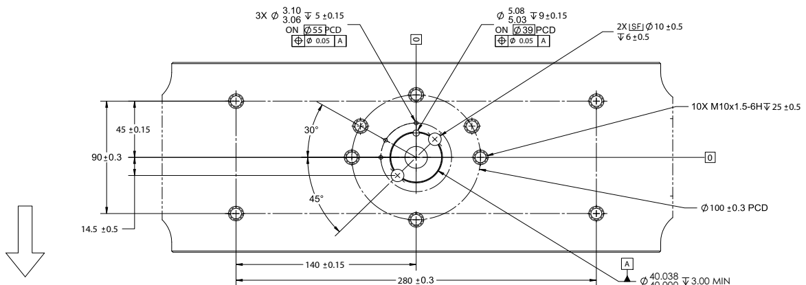
Figura 7. Vista de la parte inferior de la cruceta
