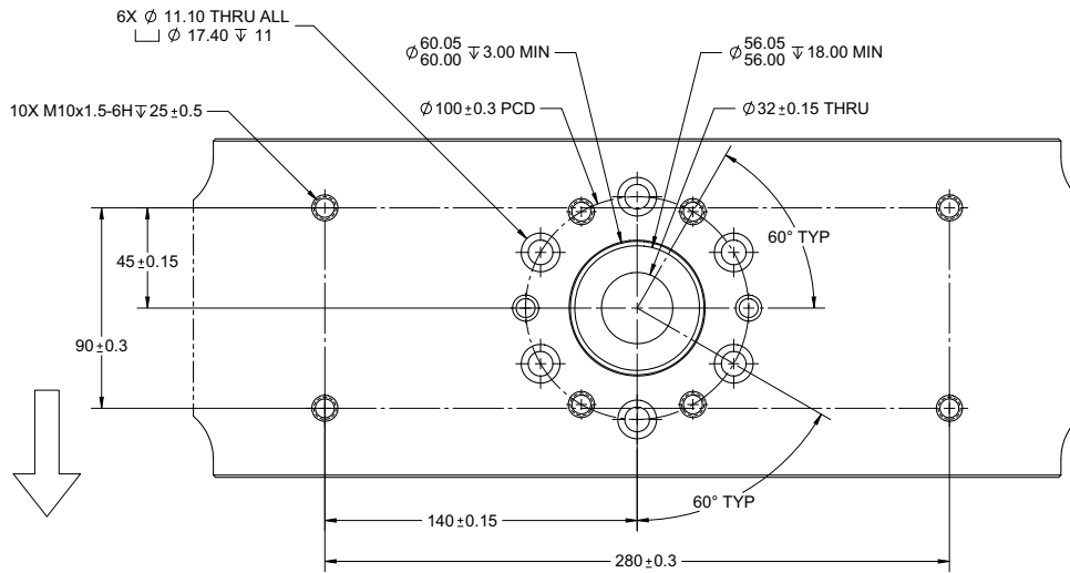
Figura 8. Vista de la parte superior de la cruceta
