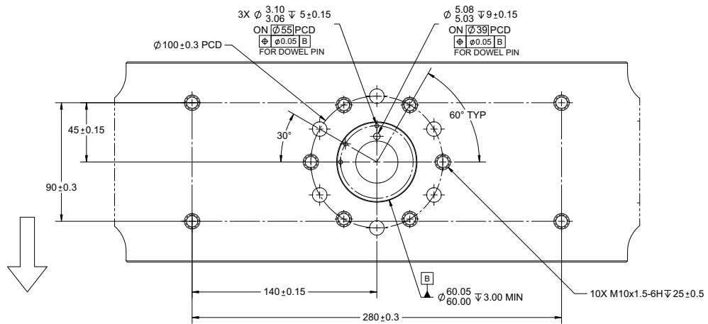
Figura 7. Vista de la parte inferior de la cruceta
