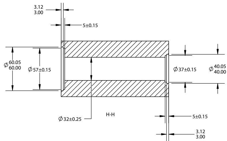
Figure 16. Vue de la section transversale H-H de la traverse
