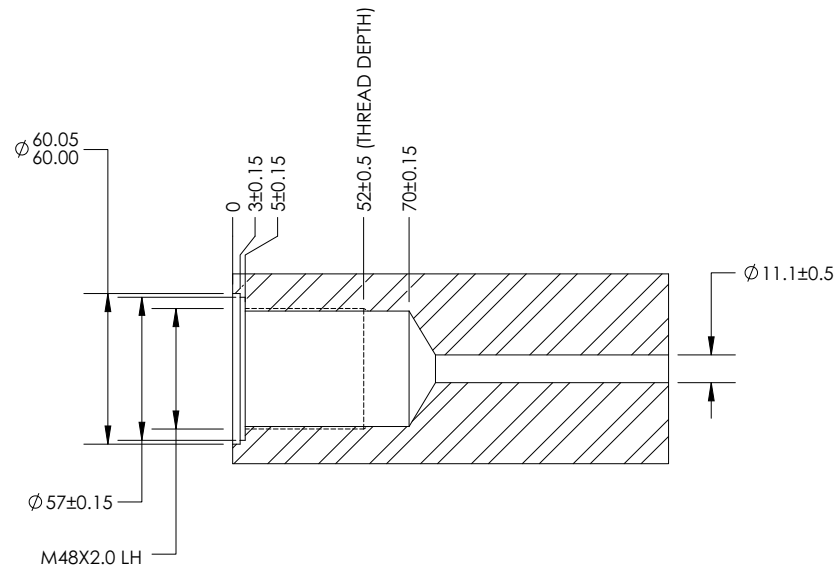
Figure 13. Vue de la section transversale G-G du socle du bâti
