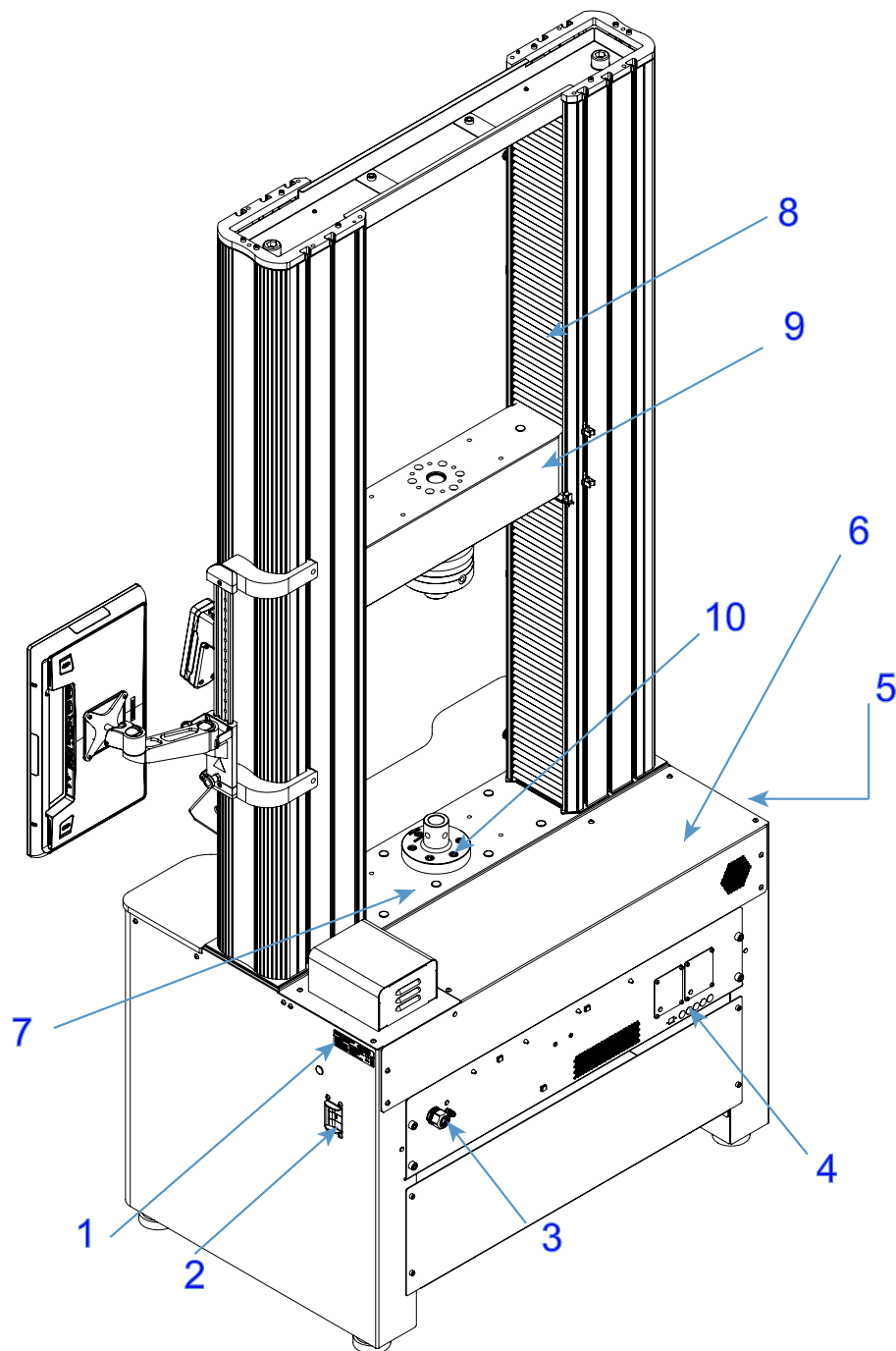
Figure 2. 68FM-100 Modèle de plancher avec Tableau de bord de l'opérateur Bluehill® - Vue de dos
