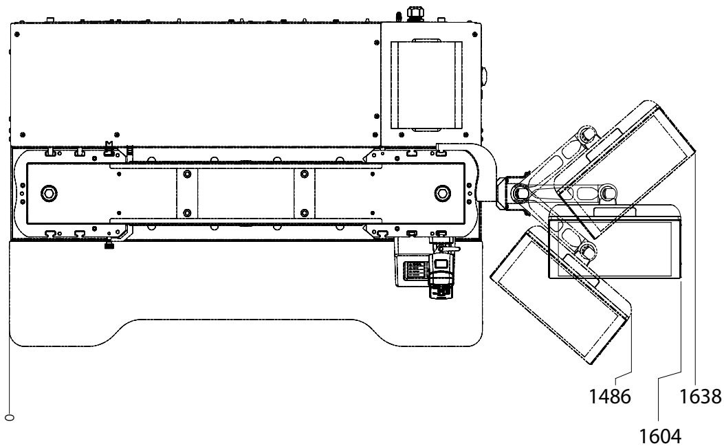
Figure 9. 68FM-100 dimensions du bâti – y compris le tableau de bord
