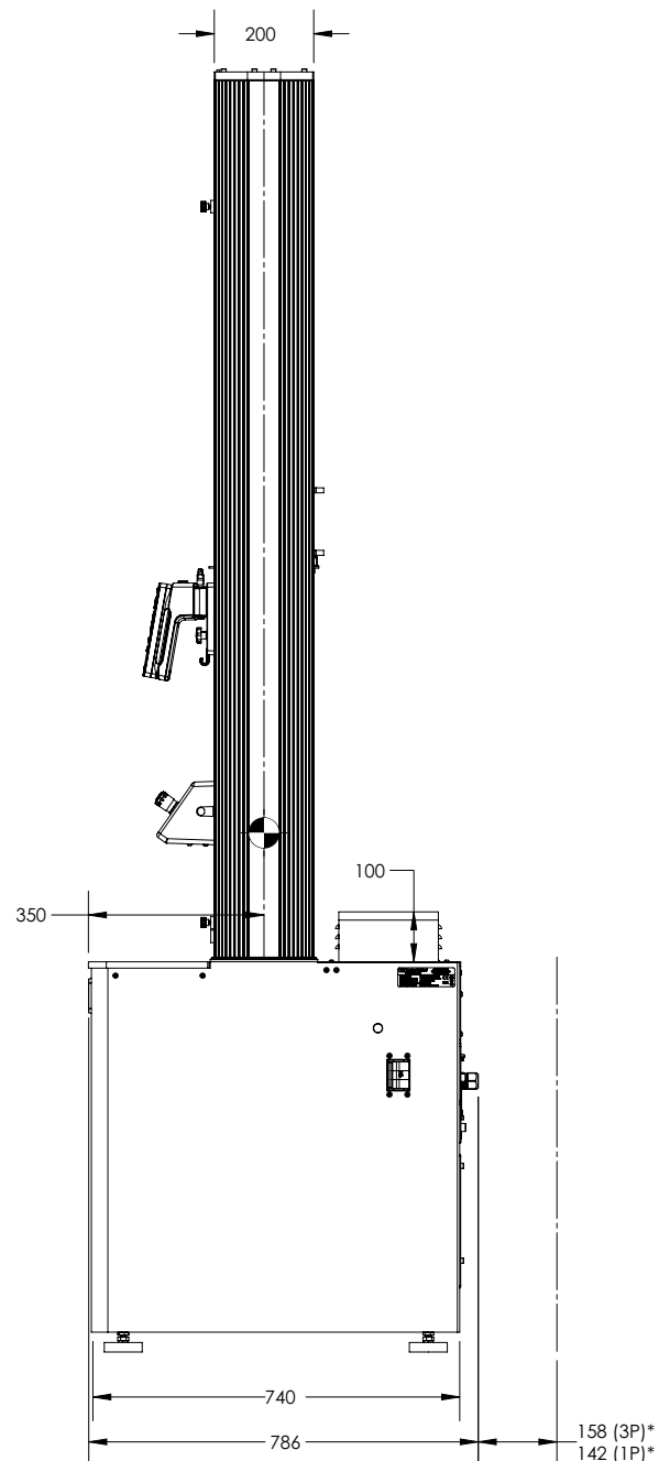
Figure 7. 68FM-100 Dimensions du bâti – vue latérale
