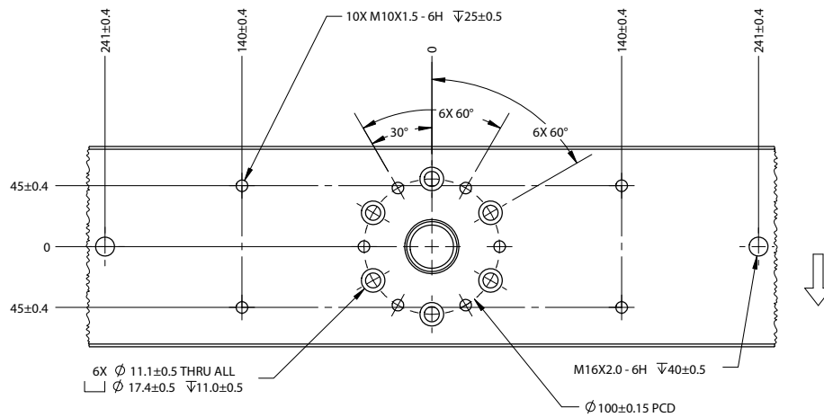
Figure 15. Vue de dessous de la traverse
