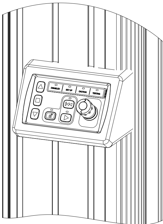
Figura 3. Vista ingrandita del pannello di controllo del telaio e del pulsante di arresto d'emergenza
