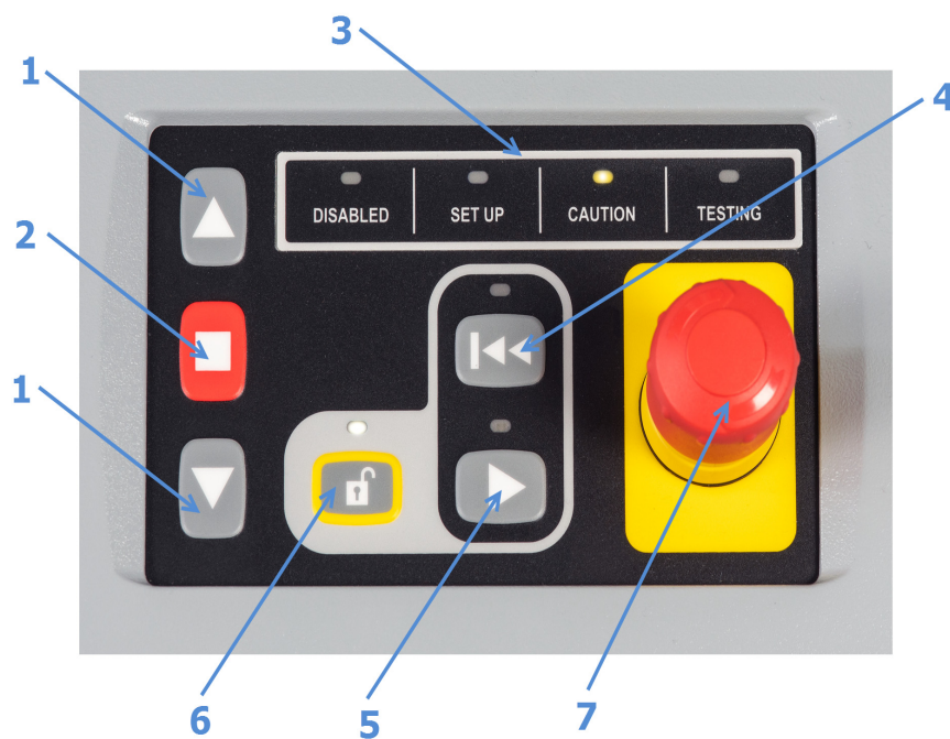
Figura 10. Pannello di controllo del telaio
