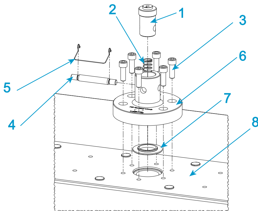
Figura 16. Adattatore di base tipo D
