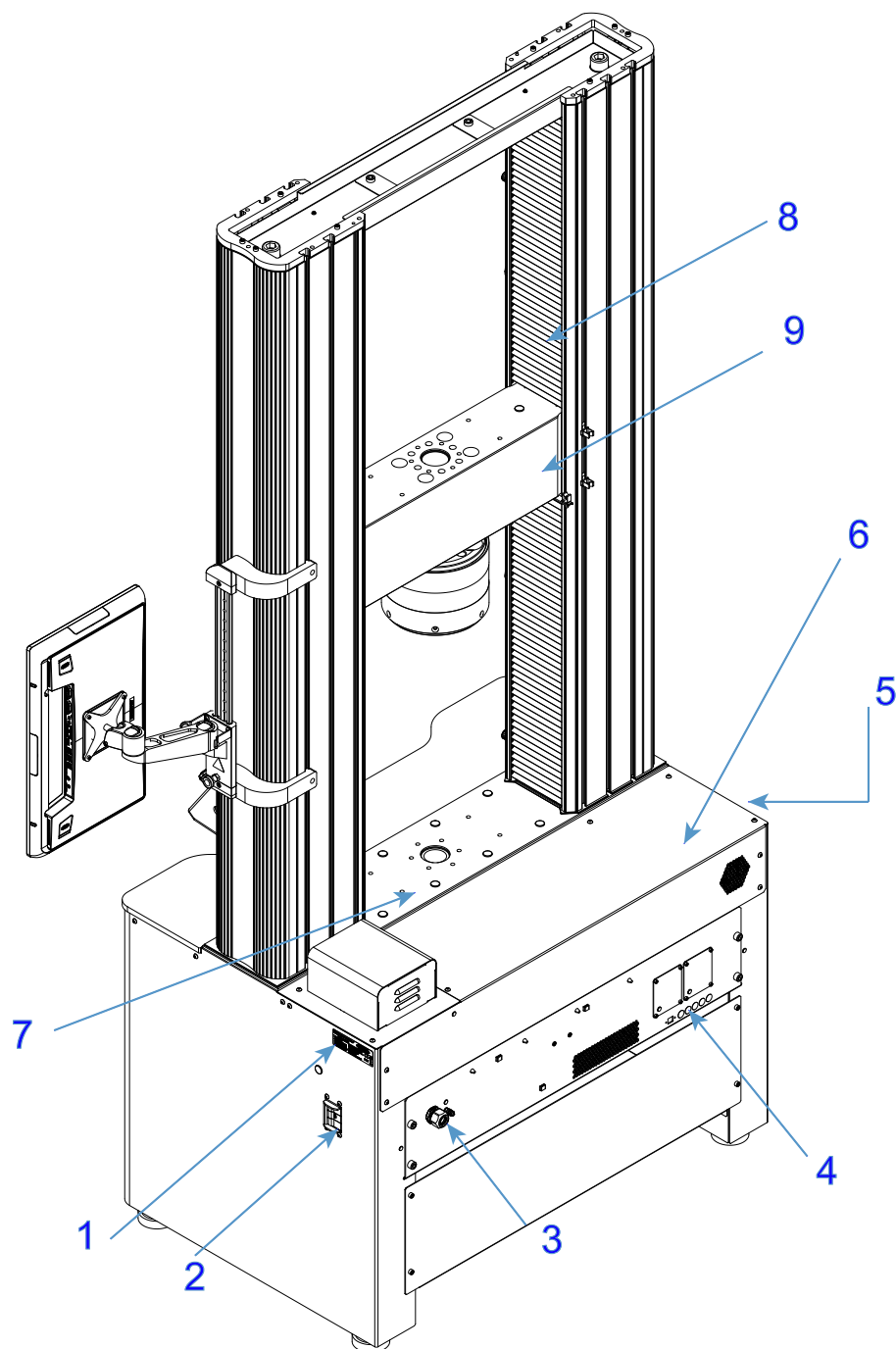
Figura 4. Modello da pavimento a doppia colonna 34FM-300 con Dashboard operatore® Bluehill - vista posteriore
