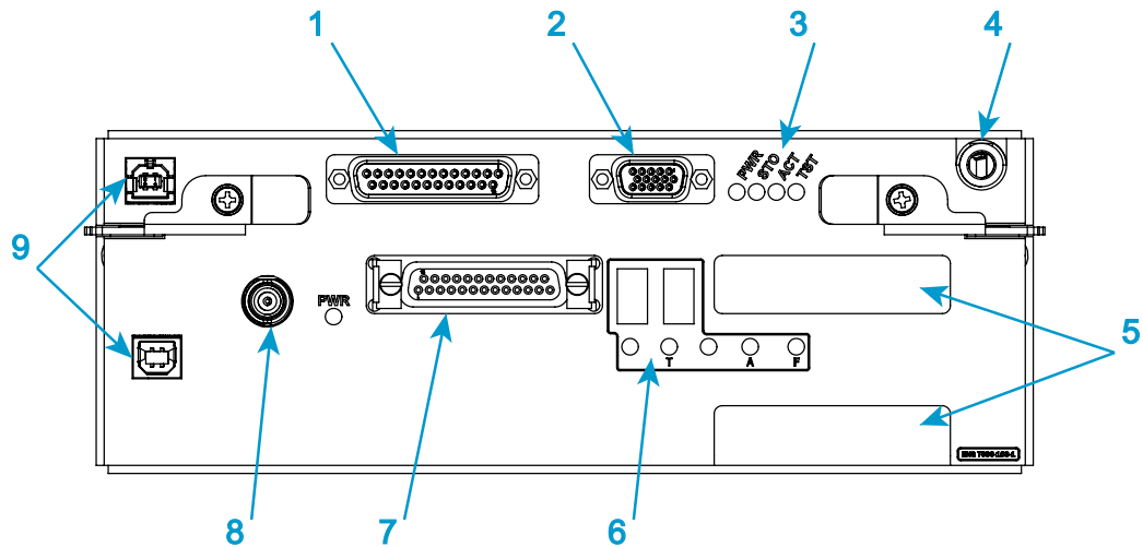
Figura 8. Dettaglio collegamenti del controller
