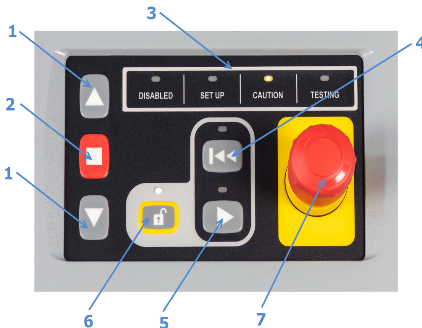
Figura 15. Pannello di controllo del telaio
