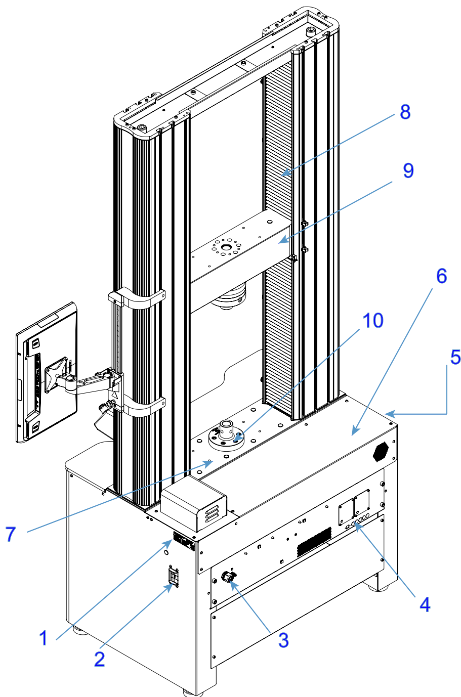
Figura 3. Modello da pavimento a doppia colonna 34FM-100 con Dashboard operatore® Bluehill - vista posteriore
