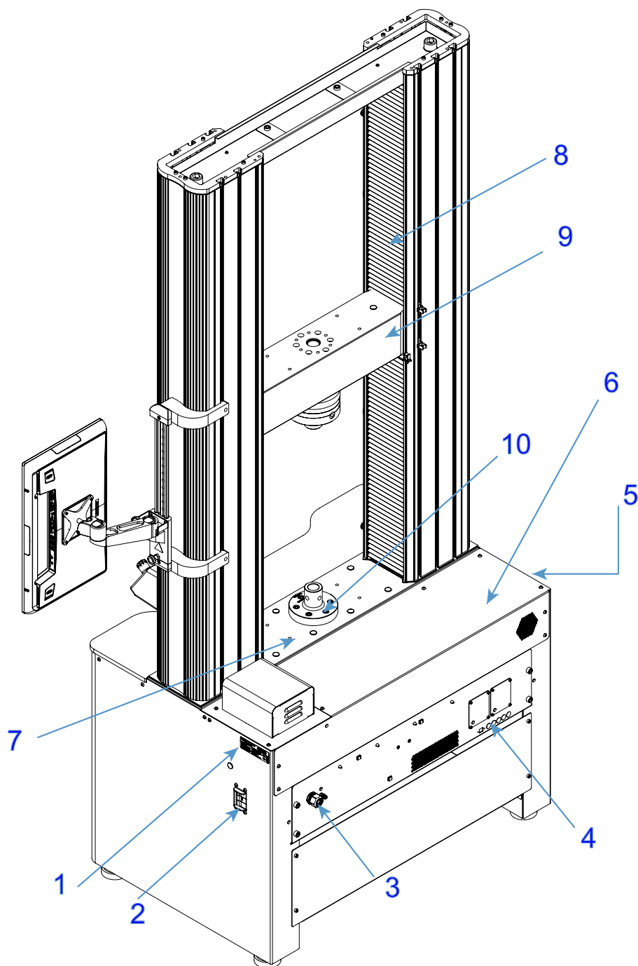
Figura 2. 34FM-100 Modello da pavimento con Dashboard operatore® Bluehill - vista posteriore
