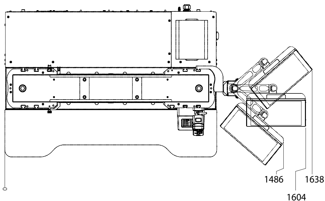
Figura 9. 34FM-100 dimensioni del telaio, inclusive di dashboard
