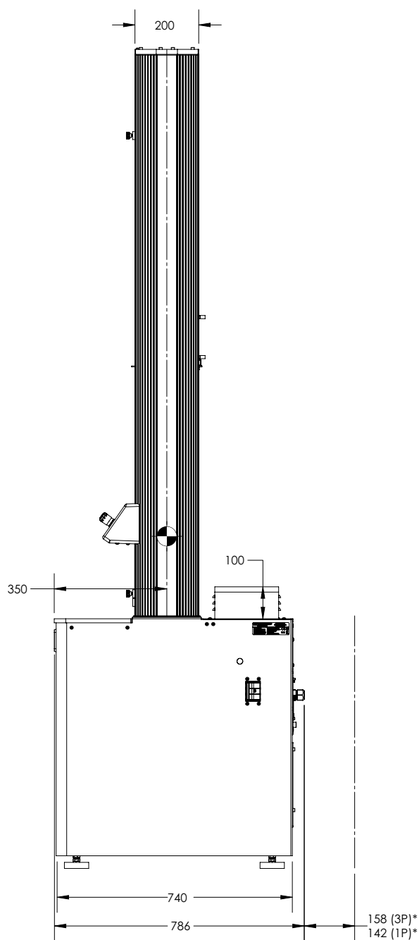
Figura 7. 34FM-100 dimensioni del telaio - vista laterale
