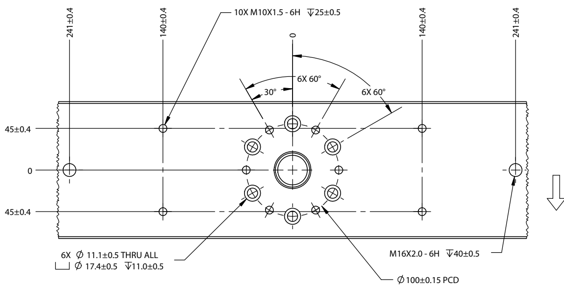
Figura 15. Vista della parte superiore della traversa
