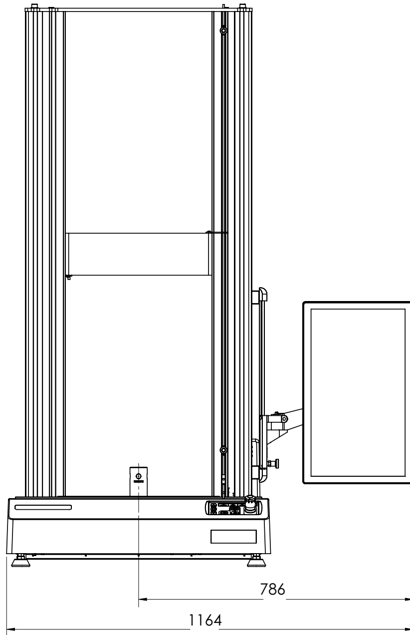
Figura 5. 34TM-10 dimensioni del telaio, inclusive di dashboard
