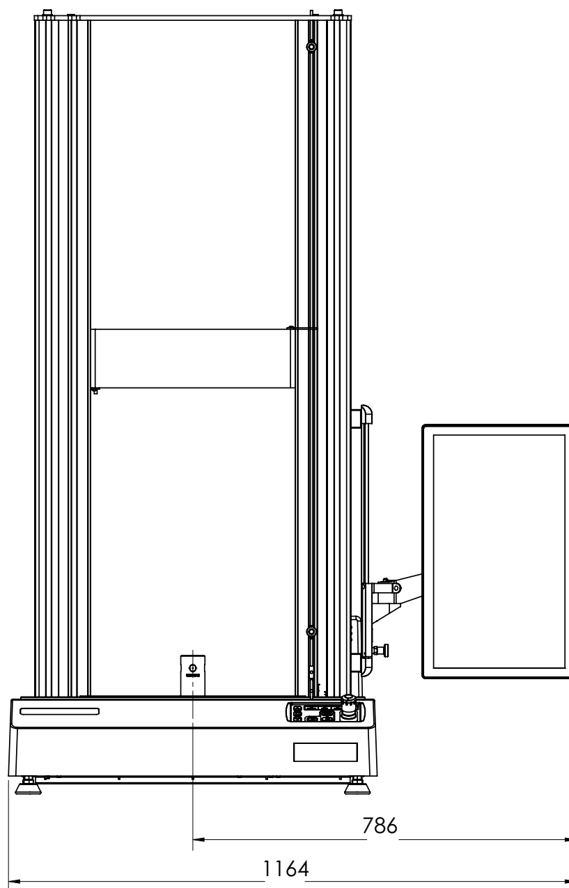
Figura 5. 34TM-30 dimensioni del telaio, inclusive di dashboard
