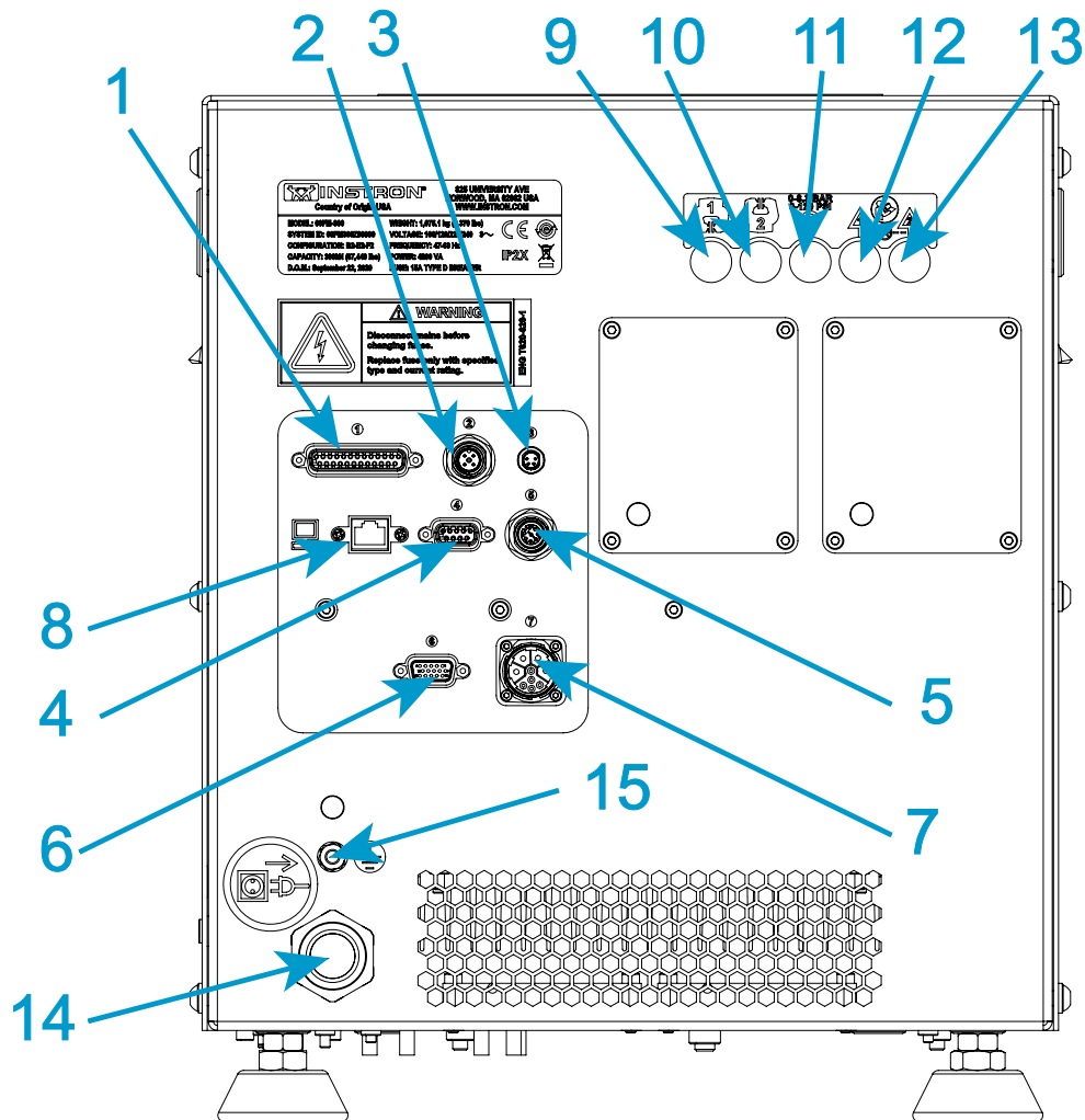
Figura 4. Dettaglio collegamenti del pannello posteriore
