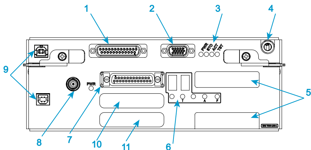
Figura 5. Dettaglio collegamenti del controller
