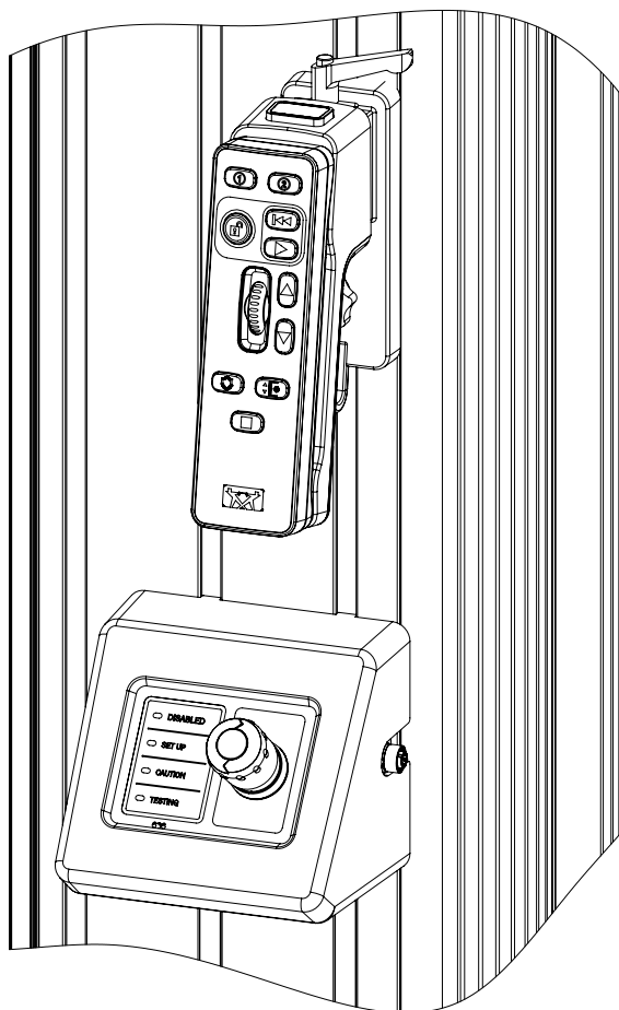
Figura 3. Visualizzazione ingrandita del pannello degli indicatori, del pulsante di arresto d'emergenza e del dispositivo di spostamento
