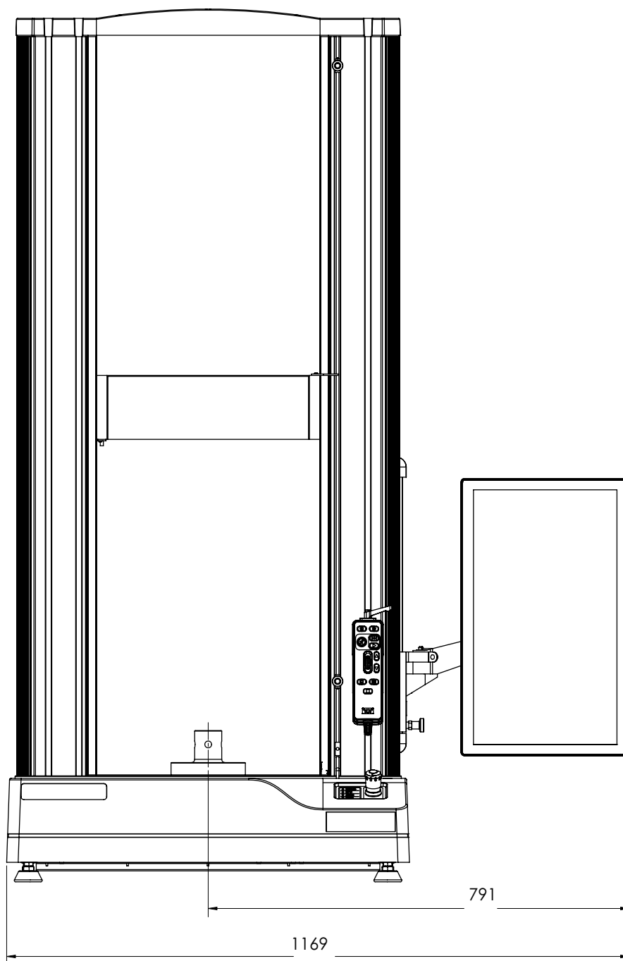
Figura 5. 68TM-10 dimensioni del telaio, inclusive di dashboard
