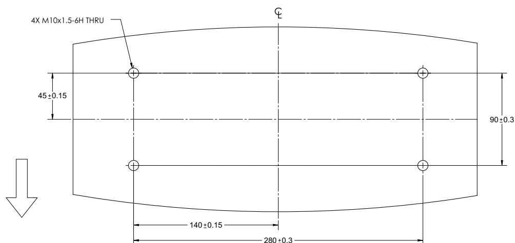
Figura 10. Vista della parte inferiore della piastra superiore
