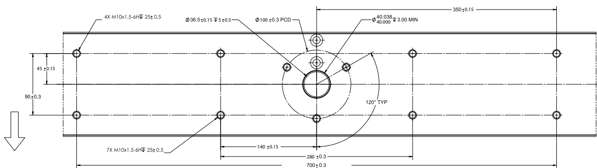
Figura 7. Vista della trave base dall'alto (solo telai dotati di larghezza supplementare)
