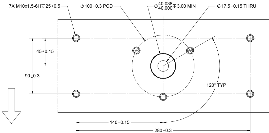
Figura 9. Vista della parte superiore della traversa
