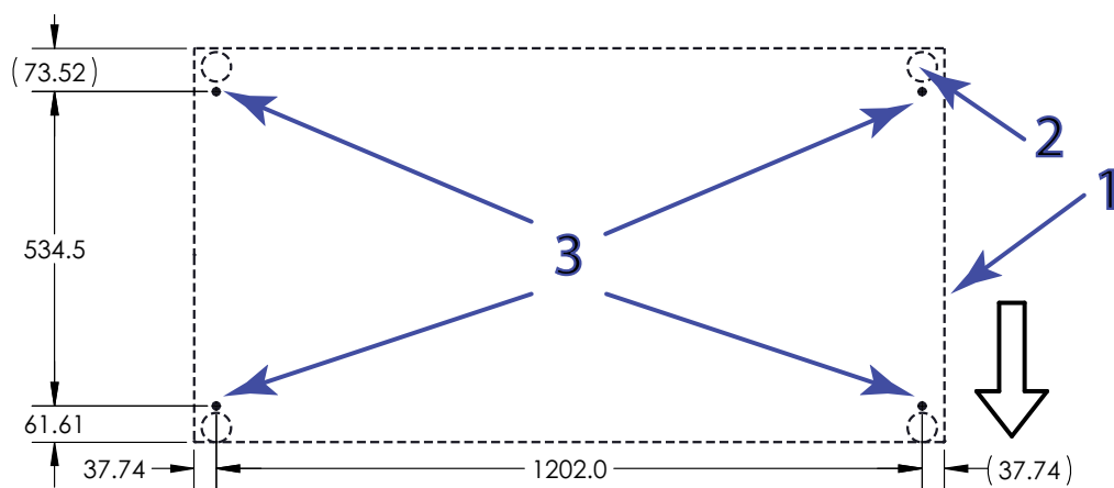
Figura 16. Posizione dei punti di ancoraggio su telaio extra largo (vista dall'alto)
