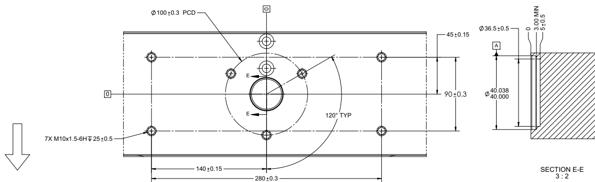
Figura 6. Vista della trave base dall'alto
