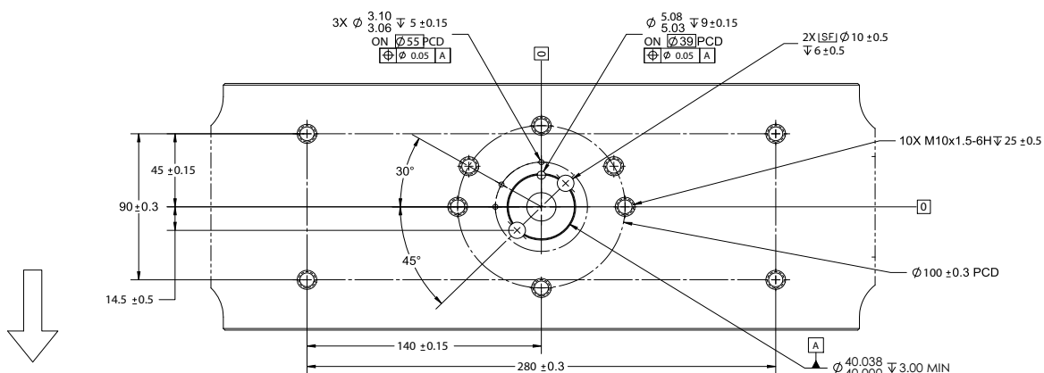
Figura 8. Vista della parte inferiore della traversa
