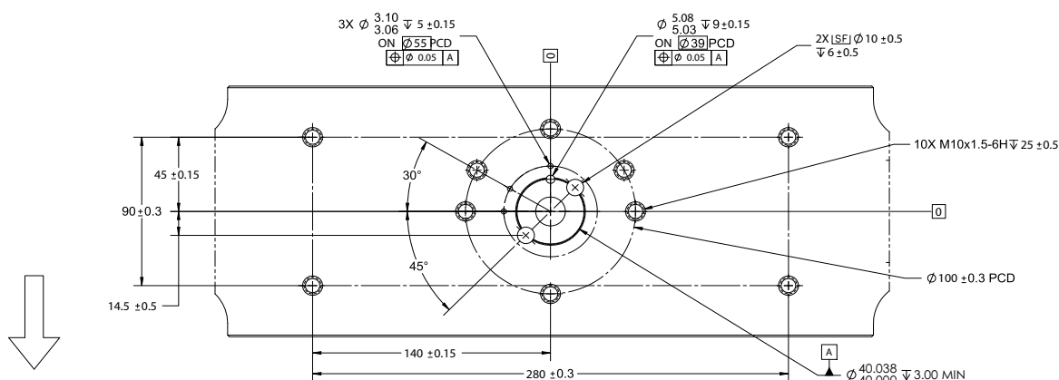
Figura 7. Vista della parte inferiore della traversa
