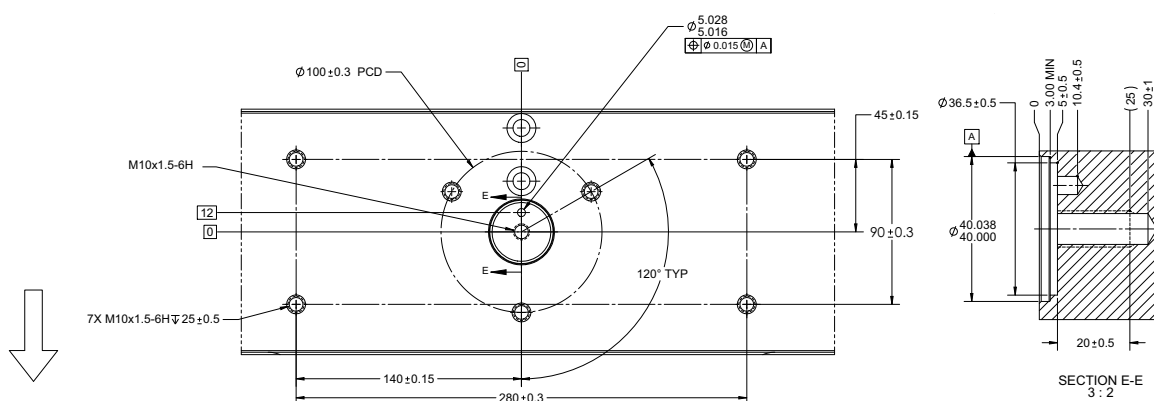
Figura 6. Vista della trave base dall'alto
