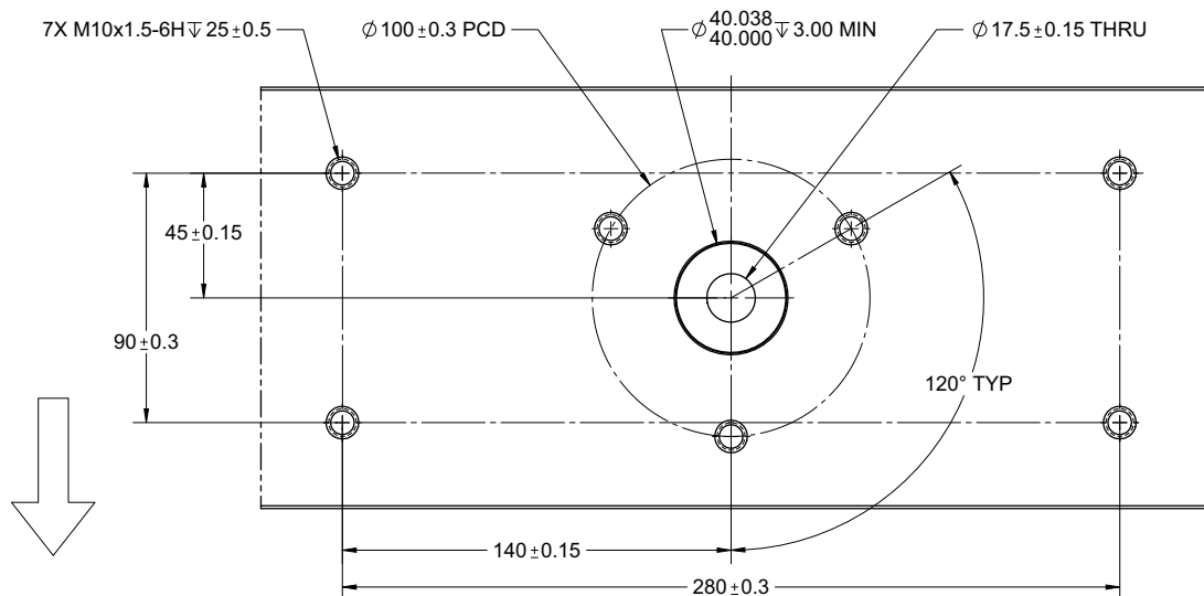
Figura 8. Vista della parte superiore della traversa
