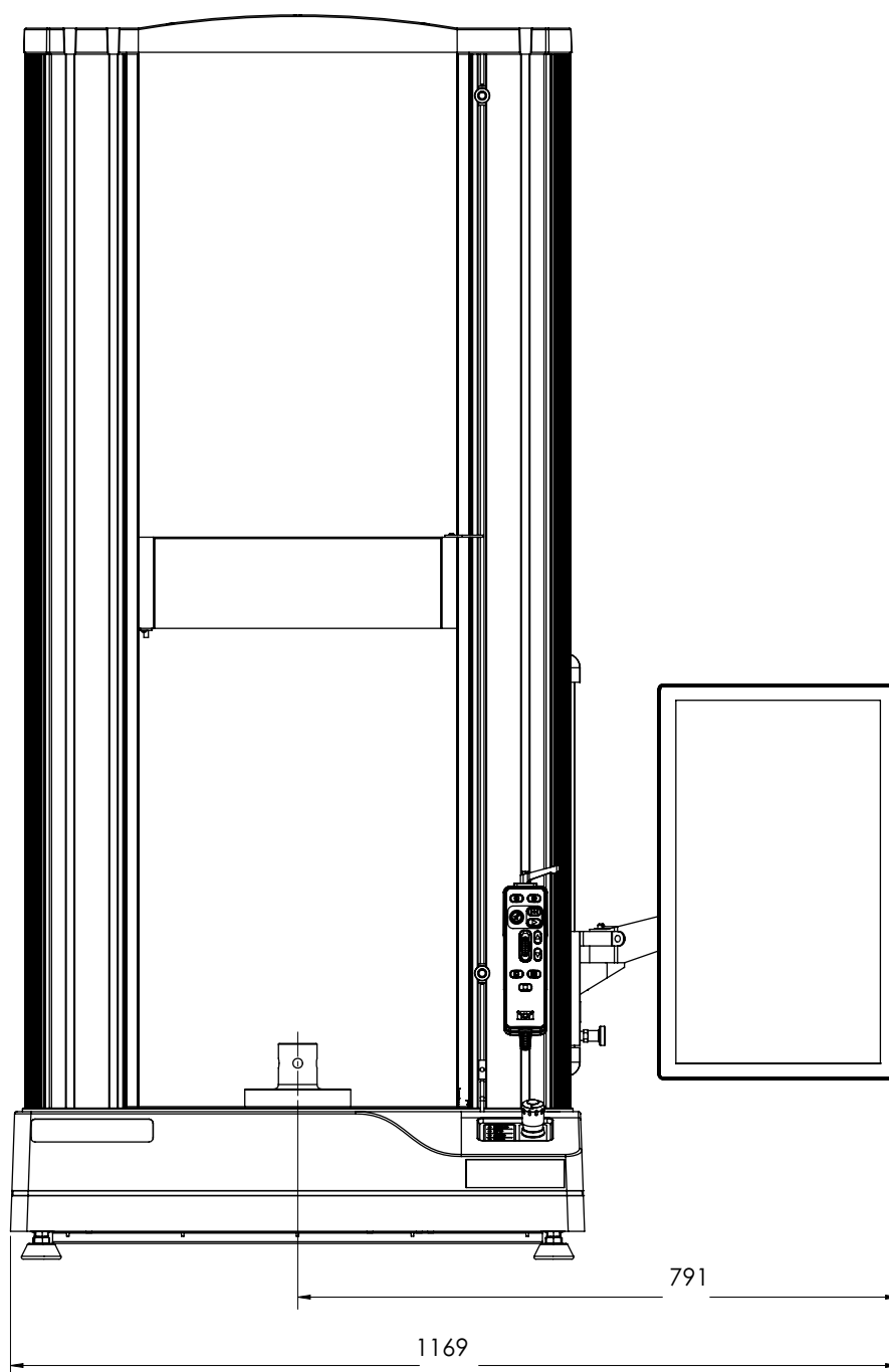
Figura 5. 68TM-50 dimensioni del telaio, inclusive di dashboard
