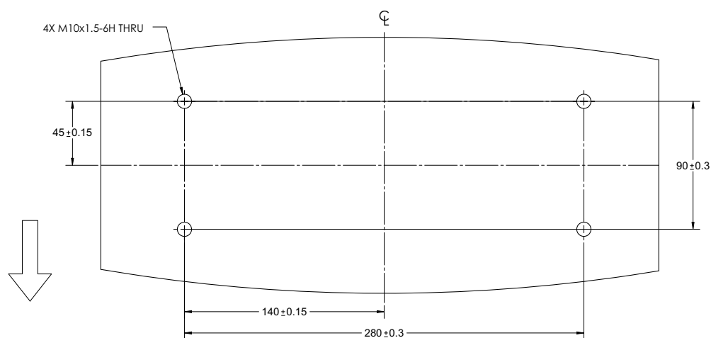
Figura 9. Vista della parte inferiore della piastra superiore
