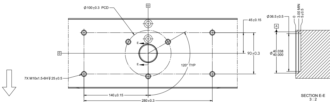
Figura 6. Vista della trave base dall'alto
