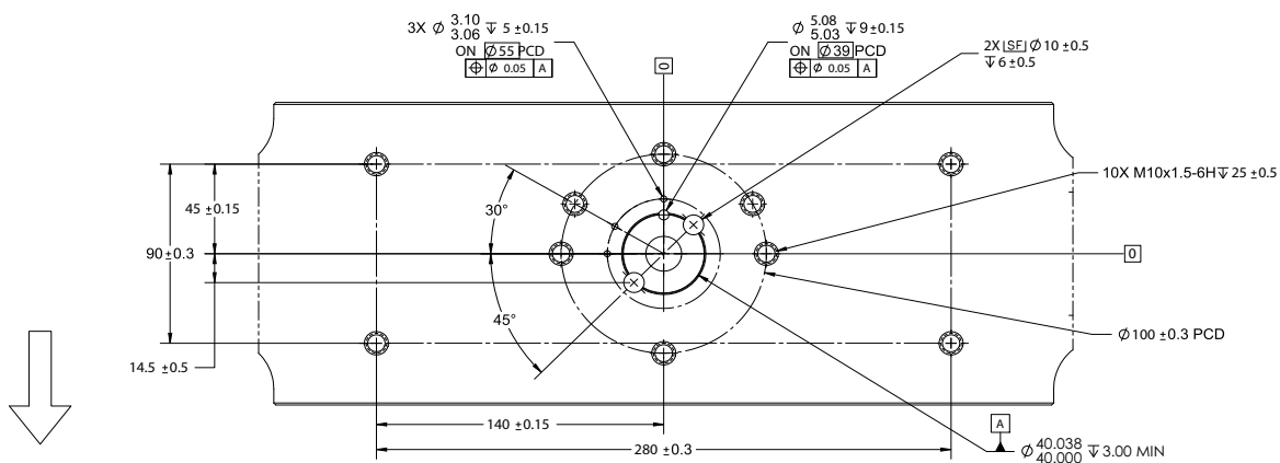
Figura 7. Vista della parte inferiore della traversa
