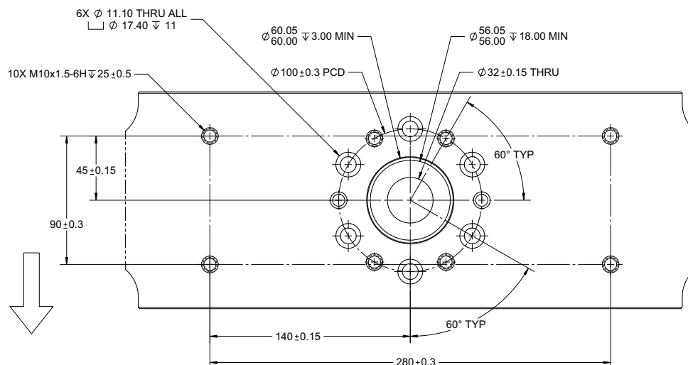
Figura 8. Vista della parte superiore della traversa
