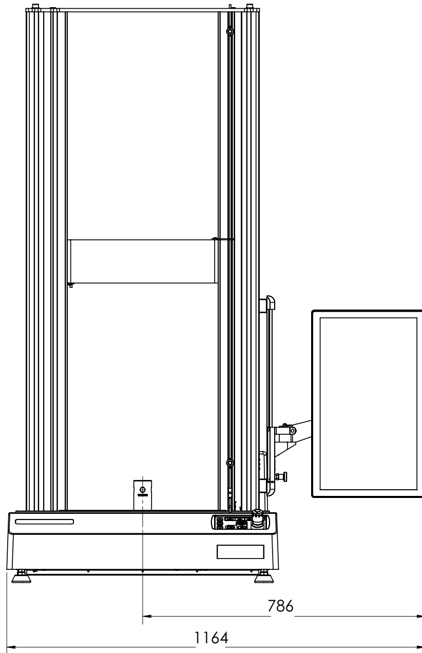
Figura 5. 34TM-5 dimensiones del bastidor, incluida la consola
