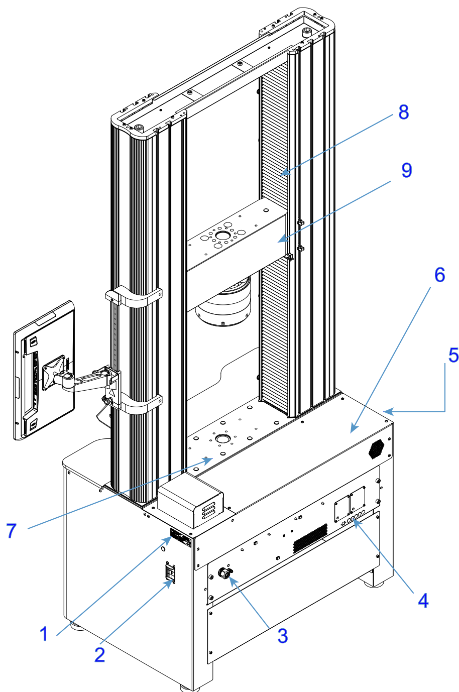
Figure 4. Modèle au sol bicolonne 34FM-300 avec Tableau de bord de l'opérateur Bluehill® – vue de dos
