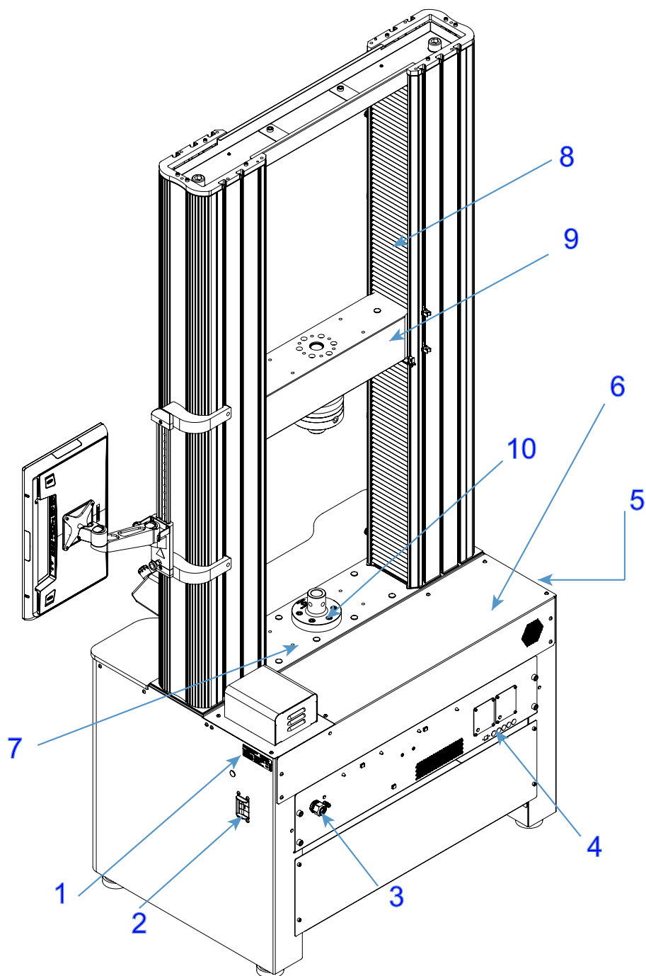
Figure 3. Modèle au sol bicolonne 34FM-100 avec Tableau de bord de l'opérateur Bluehill® – vue de dos
