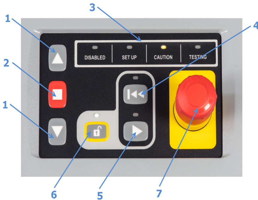
Figure 15. Panneau de commande du bâti
