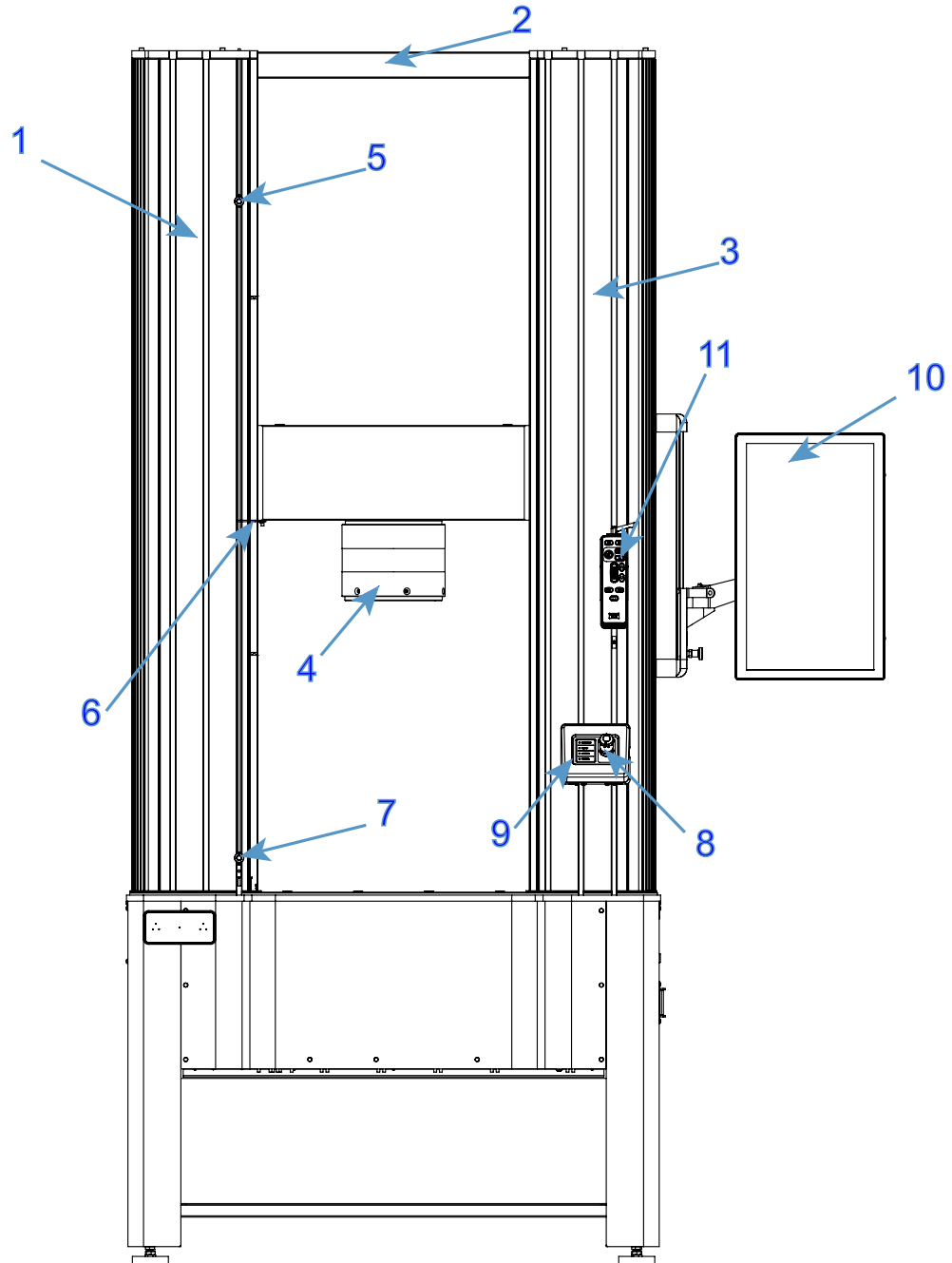
그림 1. 68FM-300 Bluehill® 작업자 대시보드( 를 ) 갖춘 바닥 모델 - 전면
