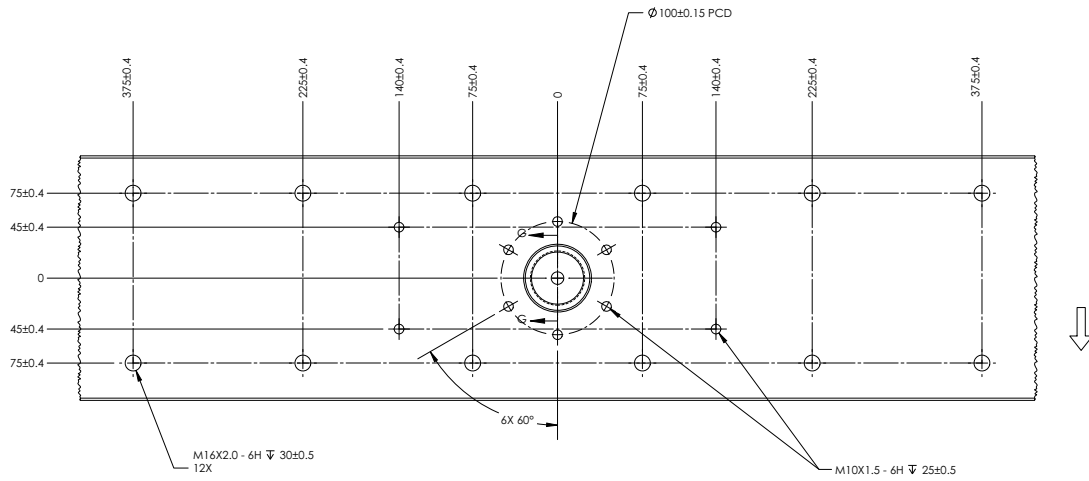
그림 13. 위에서 본 베이스 빔 ( 추가 너비 프레임만 )
