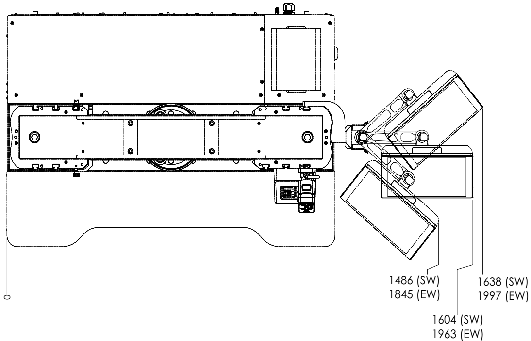
그림 9. 68FM-300 프레임 치수 - 대시보드 포함
