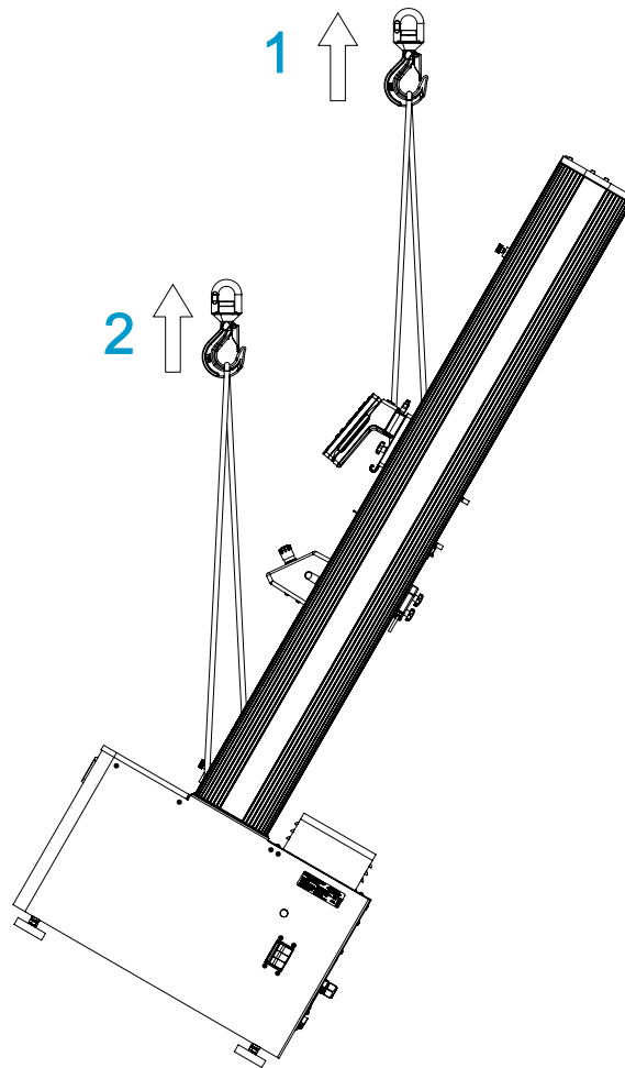
그림 19. 크레인을 이용하여 로드 프레임 세우기
