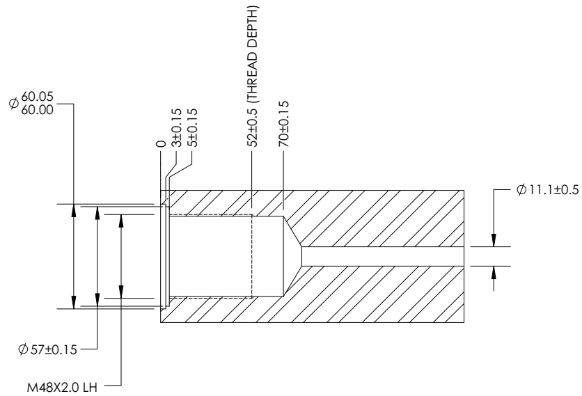
그림 14. 프레임 베이스의 G-G 단면도 보기
