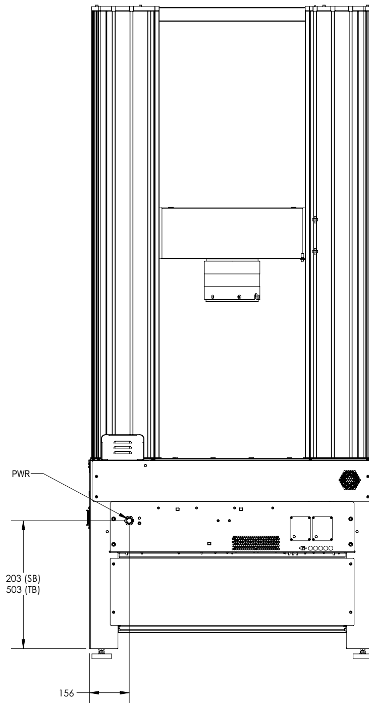
그림 8. 68FM-300 프레임 치수 - 후면
