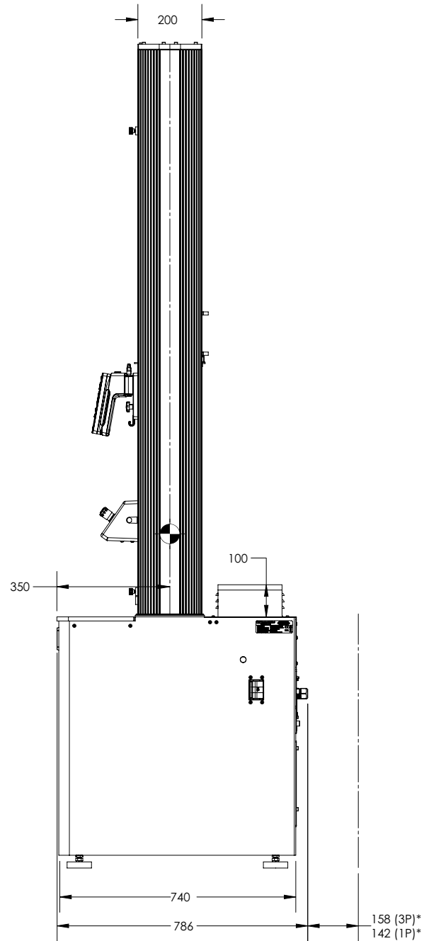
그림 7. 68FM-300 프레임 치수 - 측면
