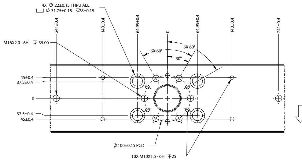
그림 16. 크로스헤드 윗면
