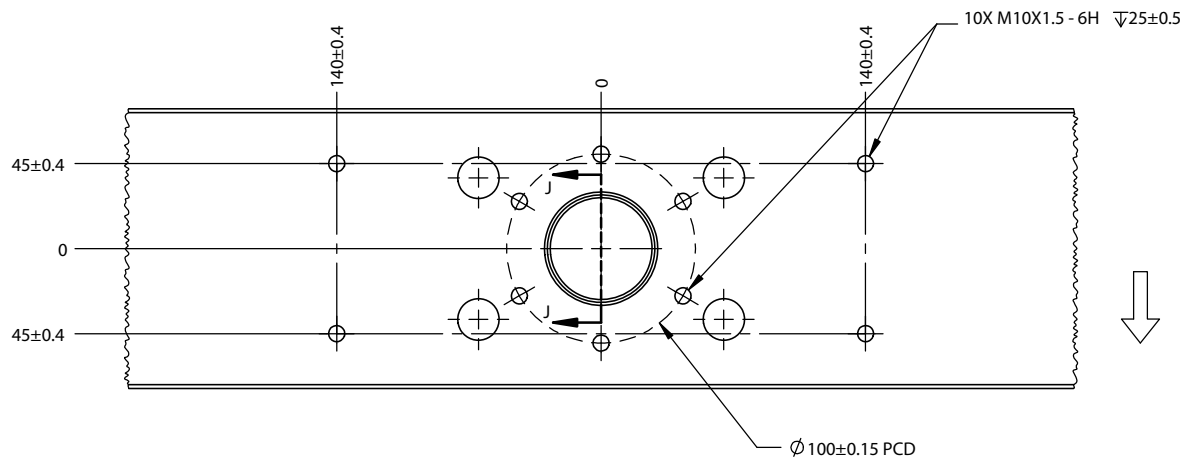
그림 15. 크로스헤드 밑면
