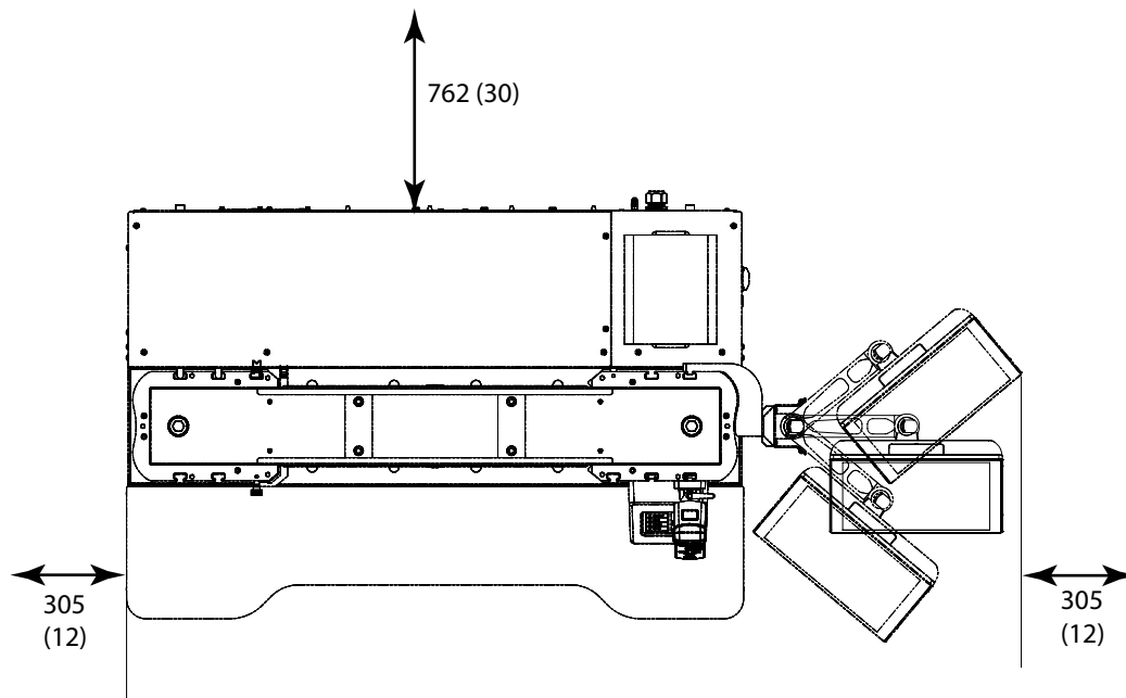
图3. 最小间隙，单位为毫米（英寸）
