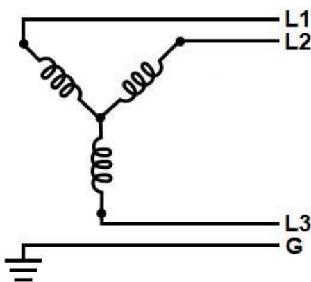
图 4.Y 形配置
