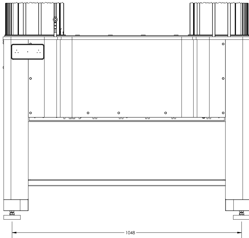
图 10. 带机架稳定器的尺寸 - 前视图
