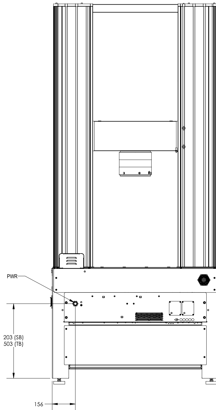
图 8.34FM-300 机架尺寸 - 背面视图
