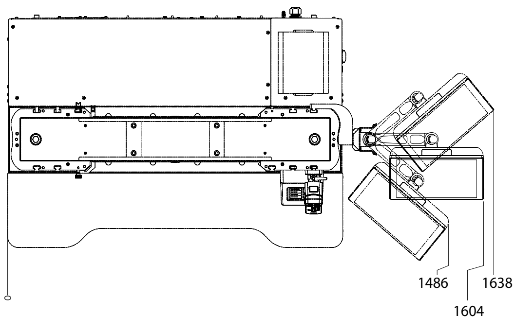
图 9.34 FM-300 机架尺寸 - 包括控制面板
