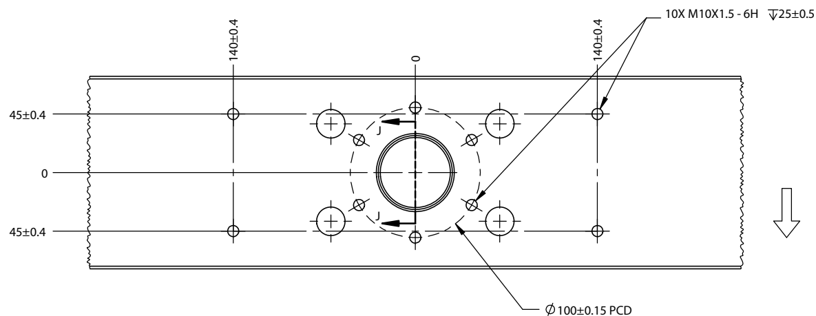
图14. 横梁下侧视图
