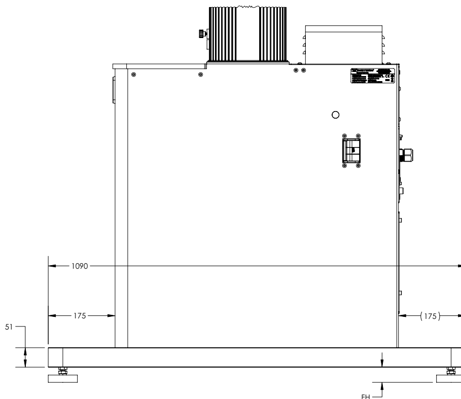
图 11. 带机架稳定器的尺寸 - 侧视图
