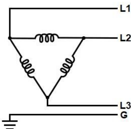
图5. 三角形配置
