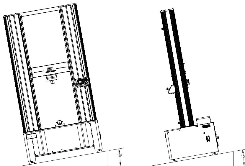
图 21. 最大倾斜角度
