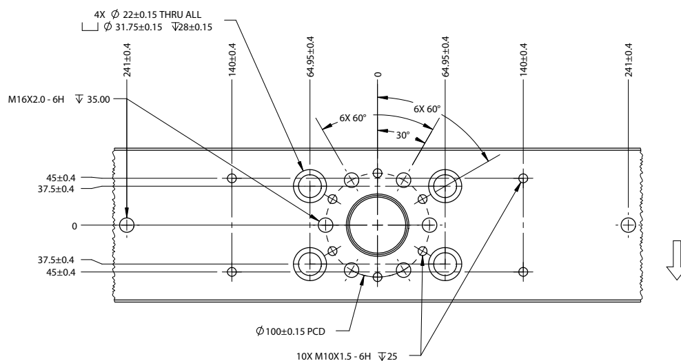
图15. 横梁上侧视图
