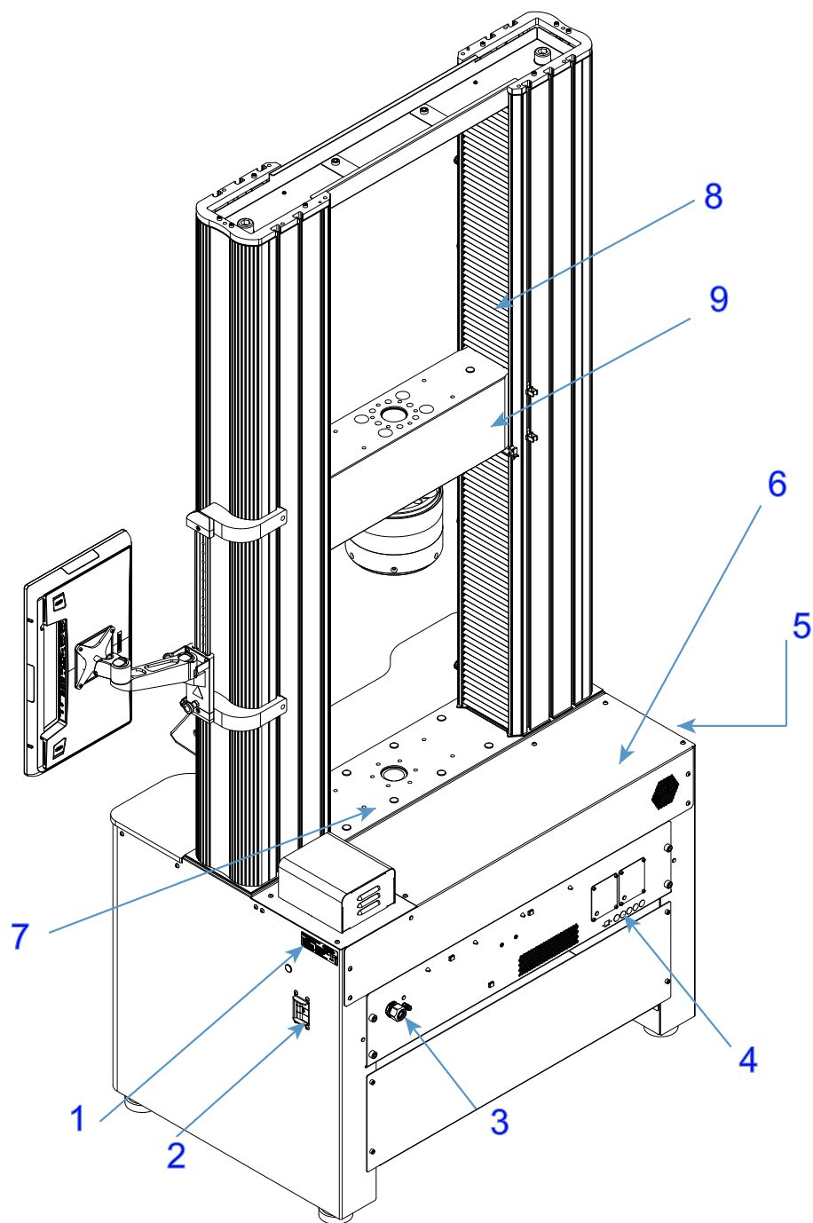
图 2.34 FM-300 含 Bluehill® 操作员控制面板 的落地式 - 背面视图
