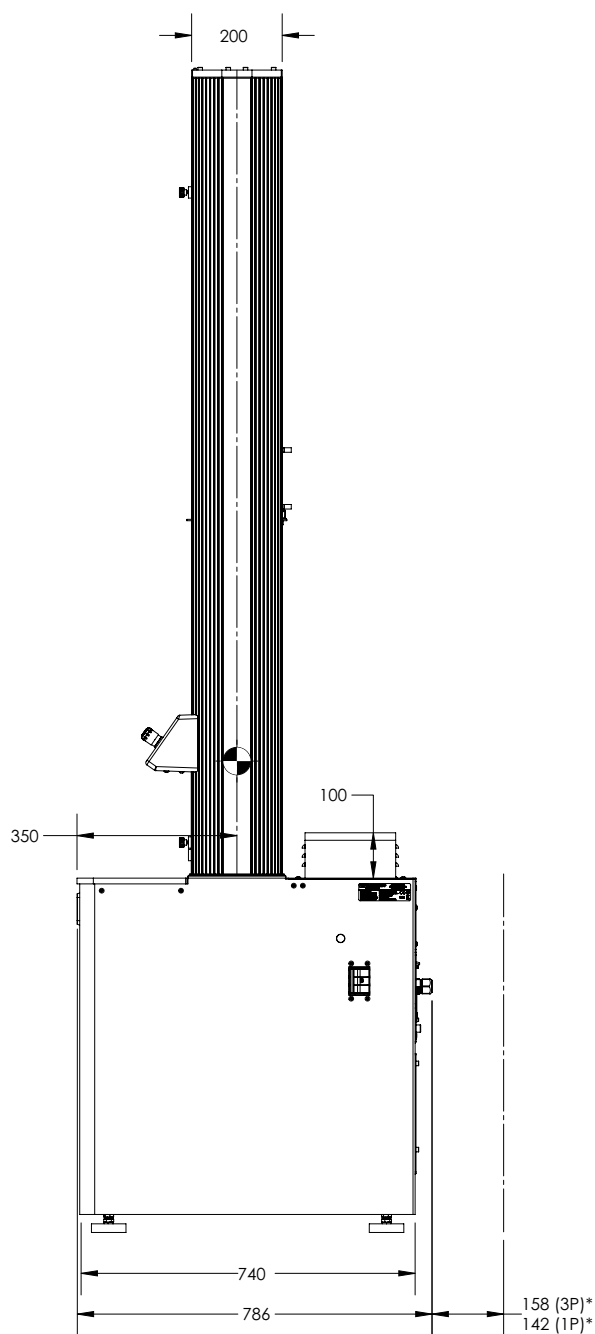
图 7.34 FM-300 机架尺寸 - 侧面视图
