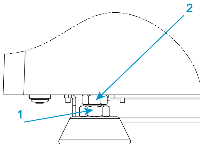
图 13. 调整水平调节支架
