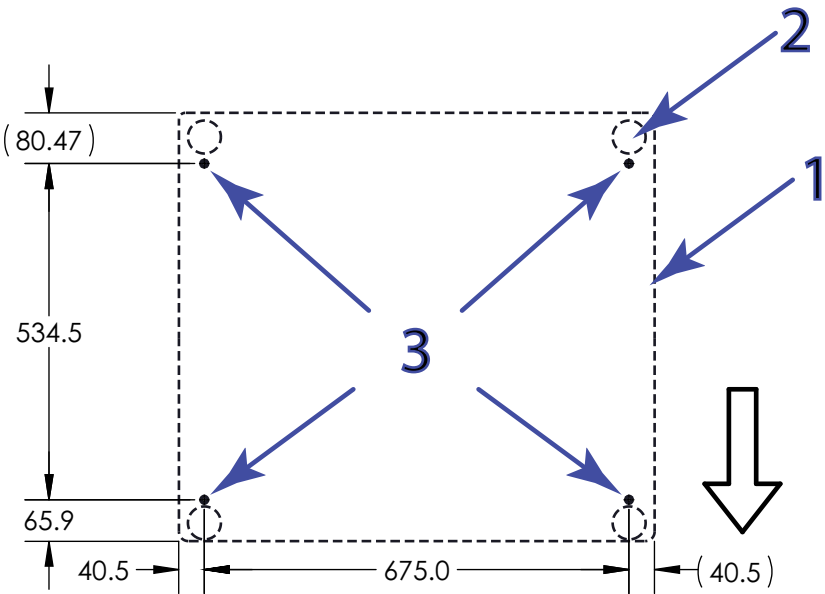
图 14. 锚固点位置（俯视）
