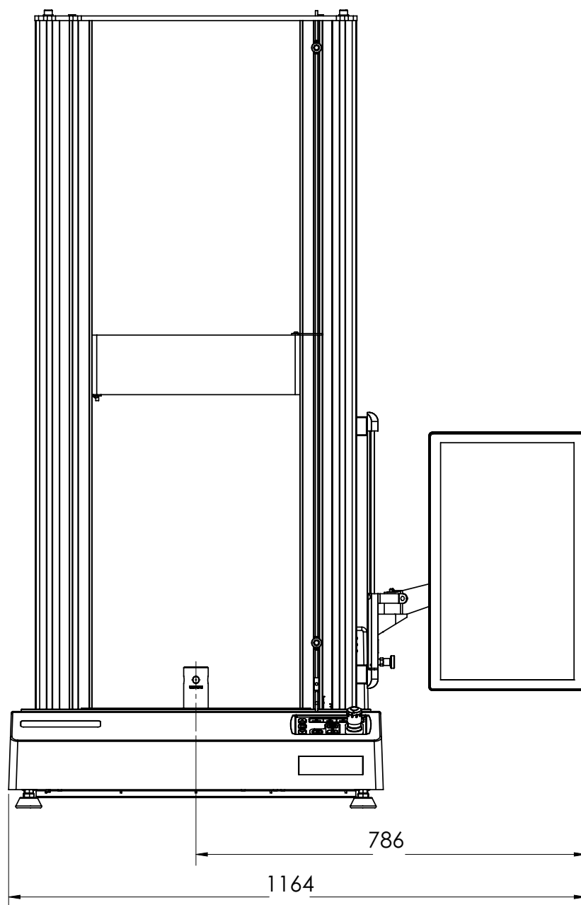
图 5.34TM-5 机架尺寸 - 包括控制面板
