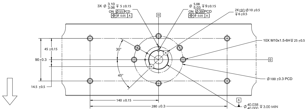
图7. 横梁下侧视图
