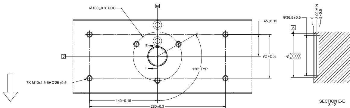
图6. 底座横梁俯视图
