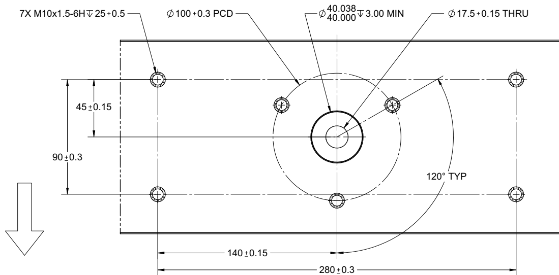
图8. 横梁上侧视图
