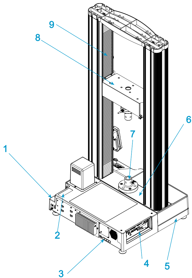
图2.6800 双立柱台式型号- 后视图
