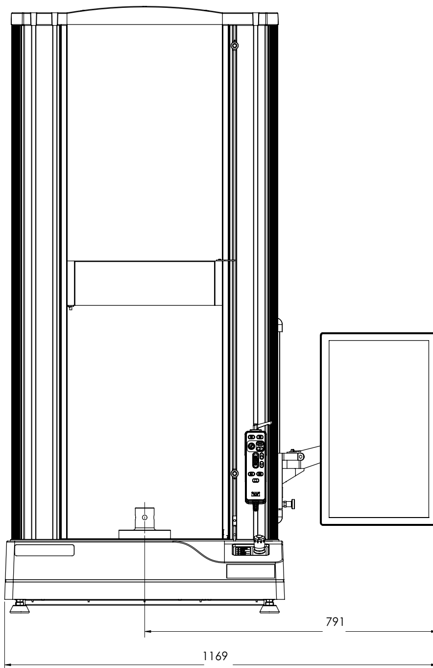
图5.68TM-50 机架尺寸- 包括控制面板
