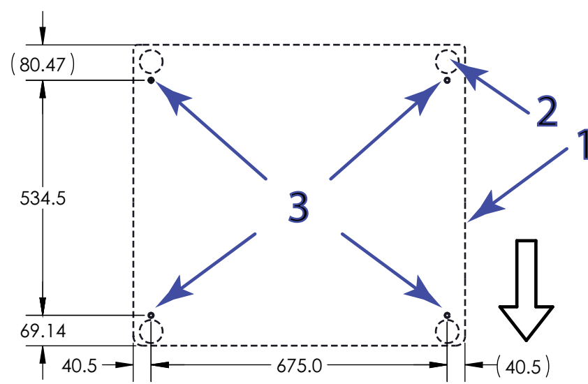
图 14. 锚固点位置（俯视）
