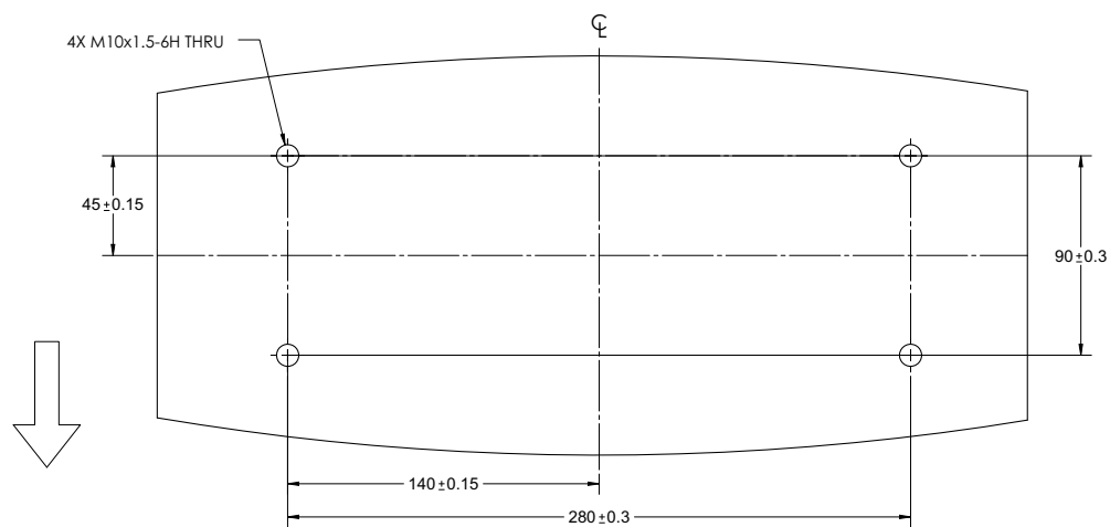
图9. 顶板下侧视图
